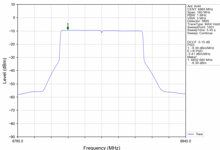
802.11ax(HEW80)_HCH_6865MHz_RU996_Left_Ant4_NTNV
