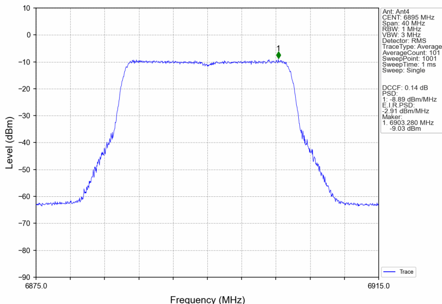
802.11ax(HEW20)_LCH_6895MHz_RU242_Left_Ant4_NTNV
