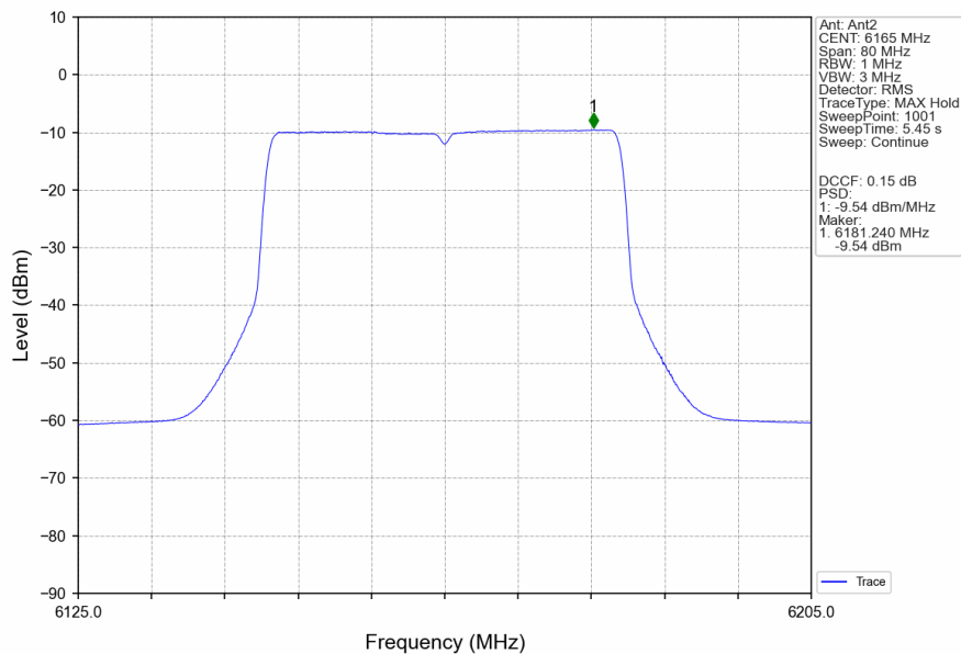
802.11ax(HEW40)_MCH_6165MHz_RU484_Left_Ant2_NTNV
