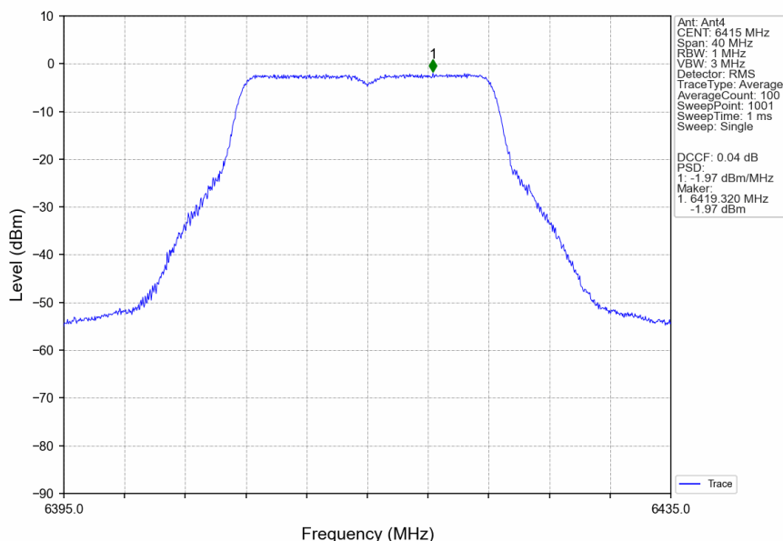
802.11a_HCH_6415MHz_Ant4_NTNV
