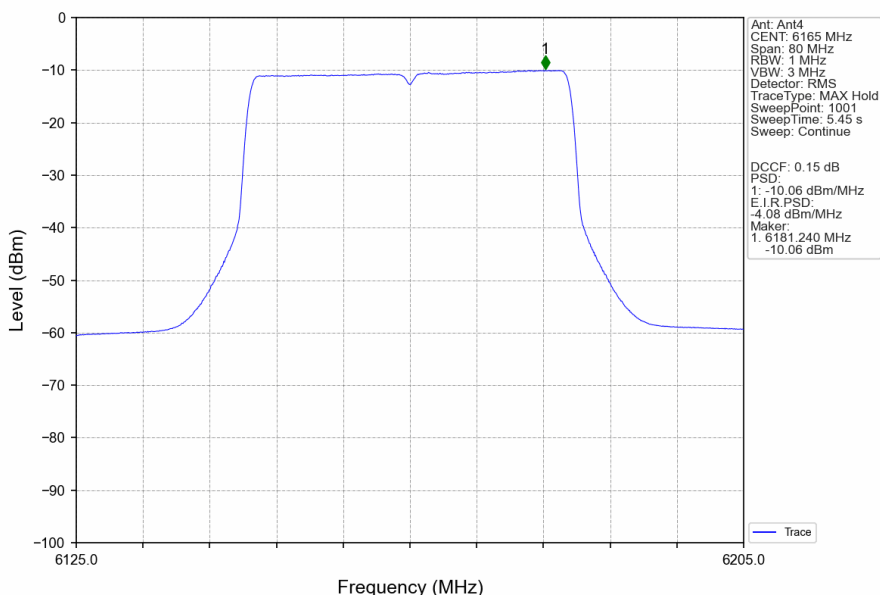
802.11ax(HEW40)_MCH_6165MHz_RU484_Left_Ant4_NTNV
