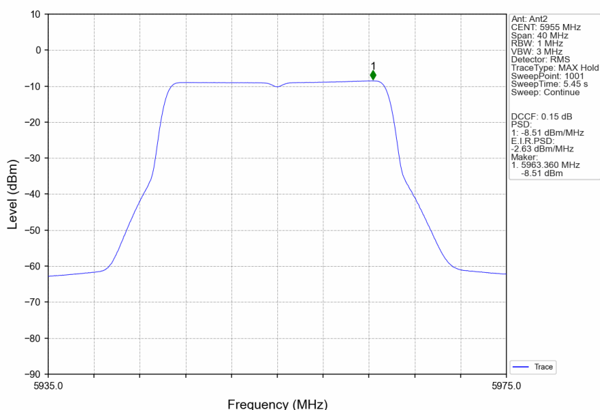
802.11ax(HEW20)_LCH_5955MHz_RU242_Left_Ant2_NTNV
