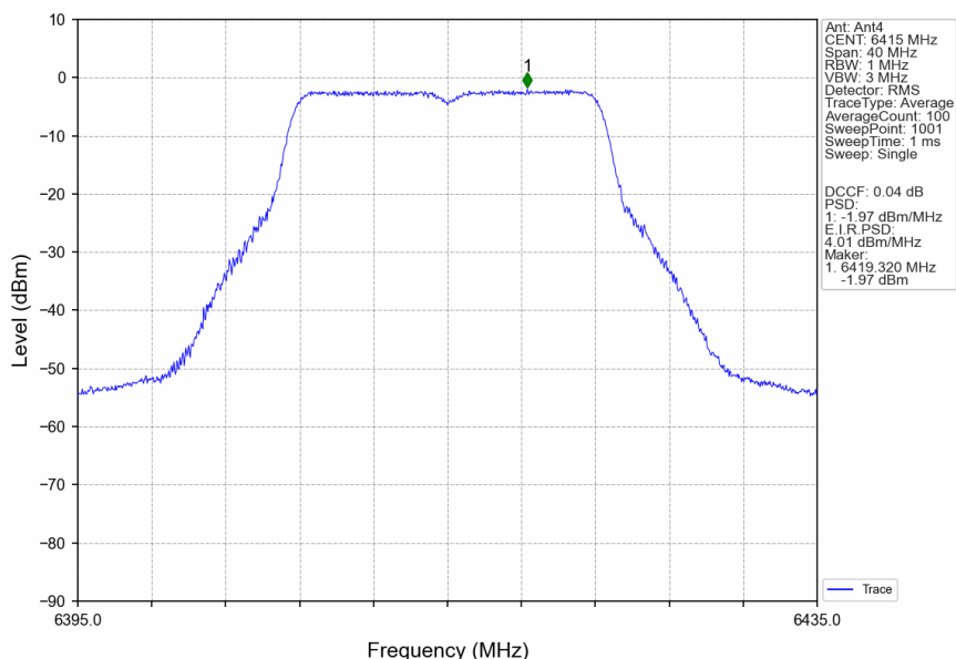
802.11a_HCH_6415MHz_Ant4_NTNV
