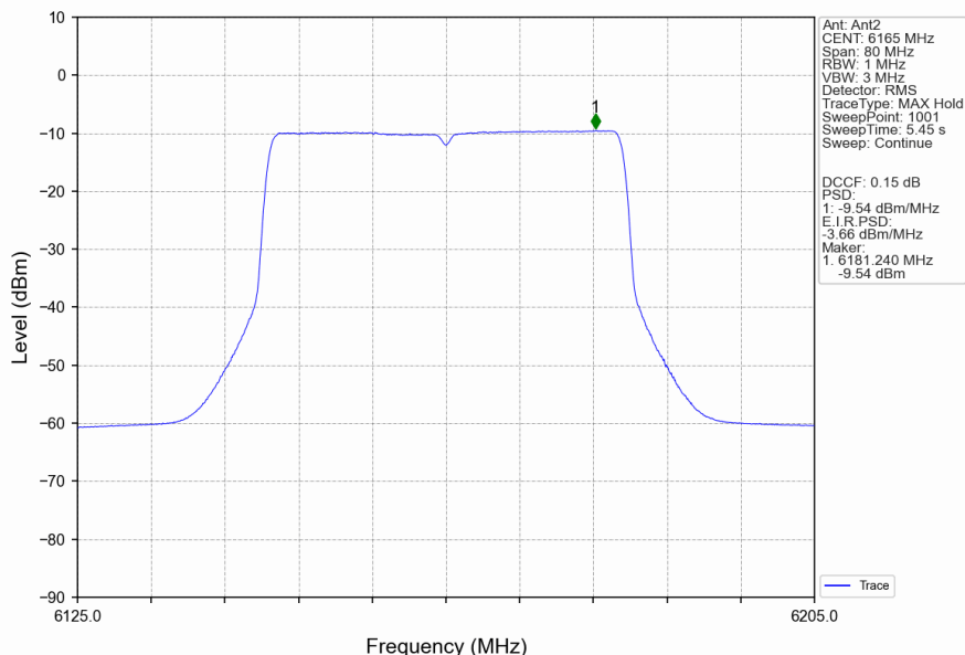
802.11ax(HEW40)_MCH_6165MHz_RU484_Left_Ant2_NTNV
