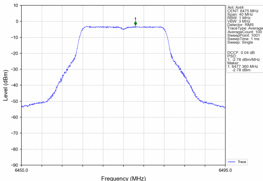
802.11a_MCH_6475MHz_Ant4_NTNV
