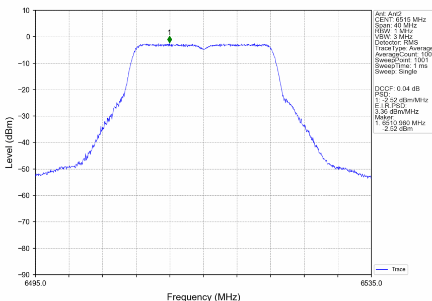
802.11a_HCH_6515MHz_Ant2_NTNV
