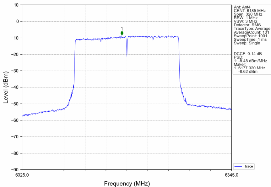
802.11be(EHT160)_MCH_6185MHz_2xRU996_Left_Ant4_NTNV
