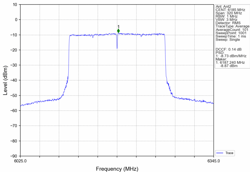
802.11be(EHT160)_MCH_6185MHz_2xRU996_Left_Ant2_NTNV
