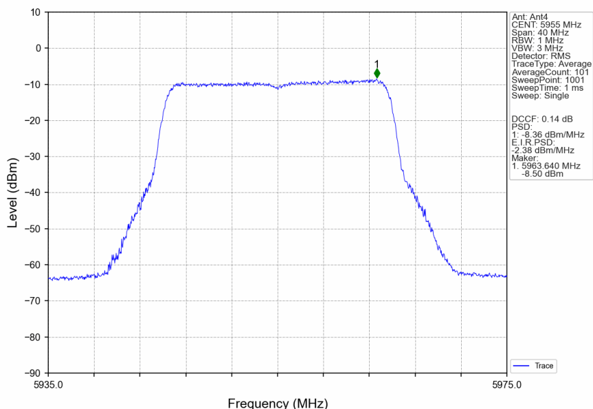
802.11be(EHT20)_LCH_5955MHz_RU242_Left_Ant4_NTNV
