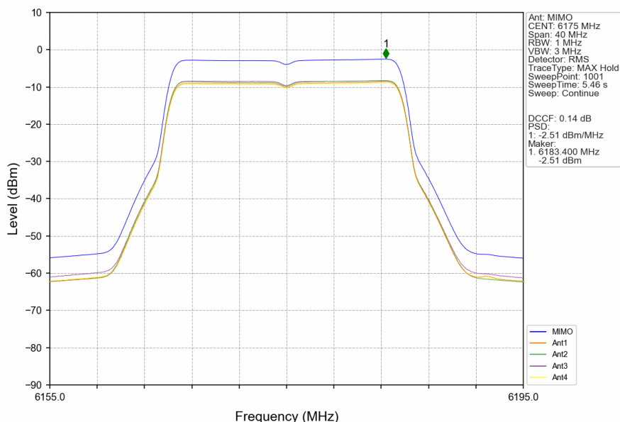
802.11be(EHT20)_MCH_6175MHz_RU242_Left_MIMO_NTNV
