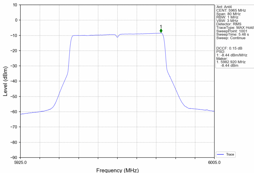
802.11be(EHT40)_LCH_5965MHz_RU484_Left_MIMO_NTNV
