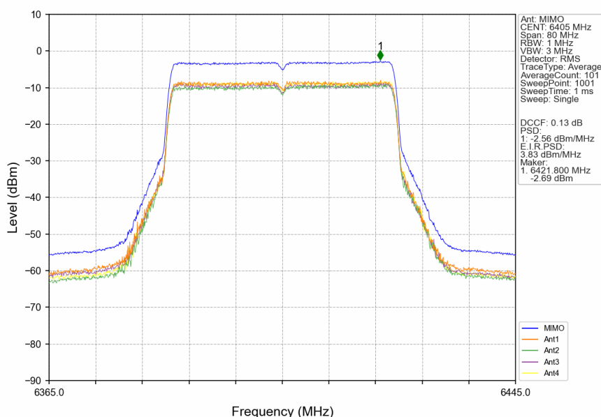
802.11be(EHT40)_HCH_6405MHz_RU484_Left_MIMO_NTNV
