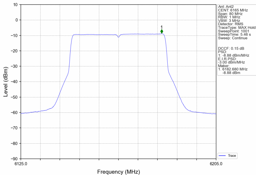
802.11be(EHT40)_MCH_6165MHz_RU484_Left_Ant2_NTNV
