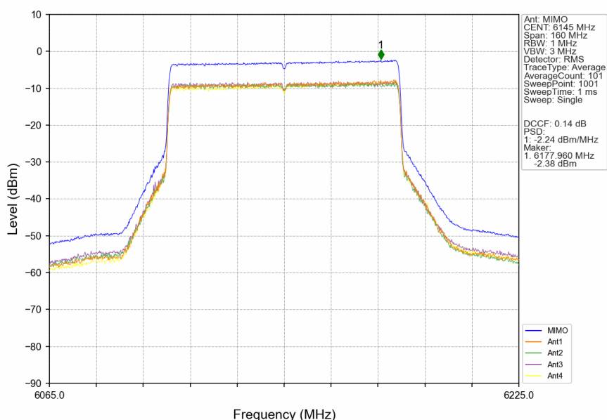
802.11be(EHT80)_MCH_6145MHz_RU996_Left_MIMO_NTNV
