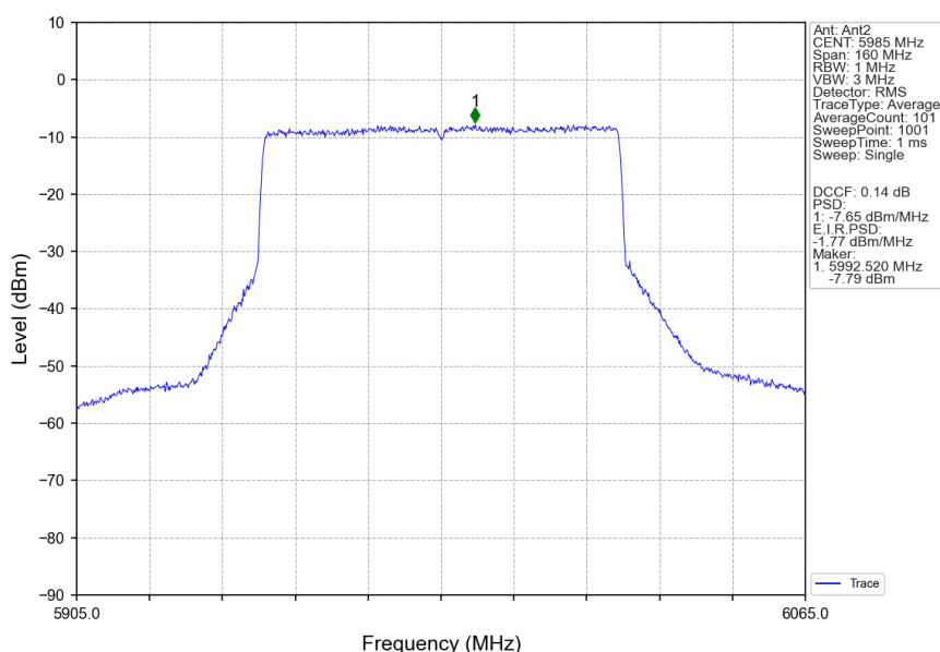
802.11be(EHT80)_LCH_5985MHz_RU996_Left_Ant2_NTNV
