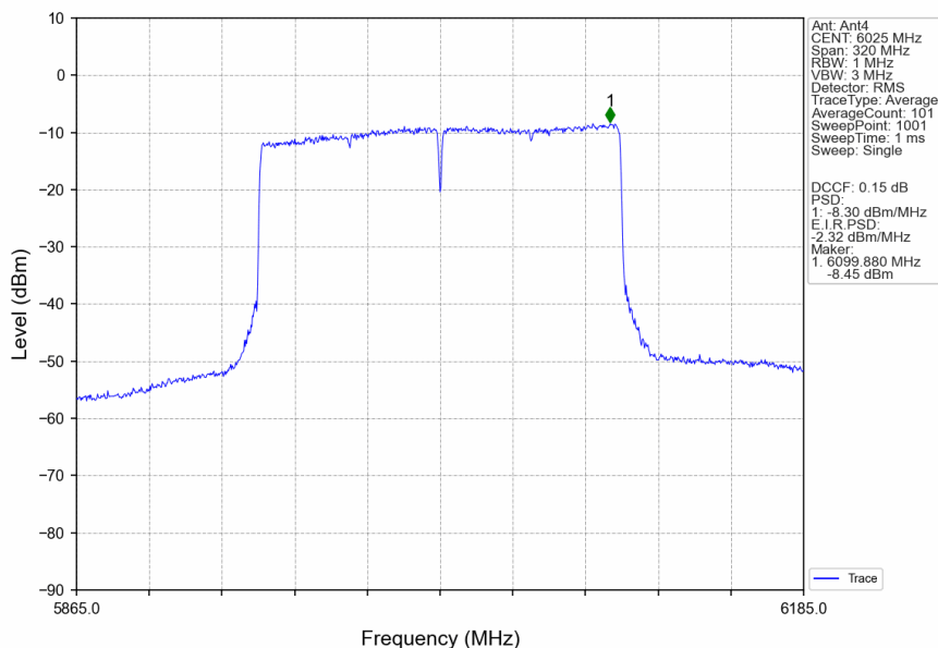
802.11be(EHT160)_LCH_6025MHz_2xRU996_Left_MIMO_NTNV
