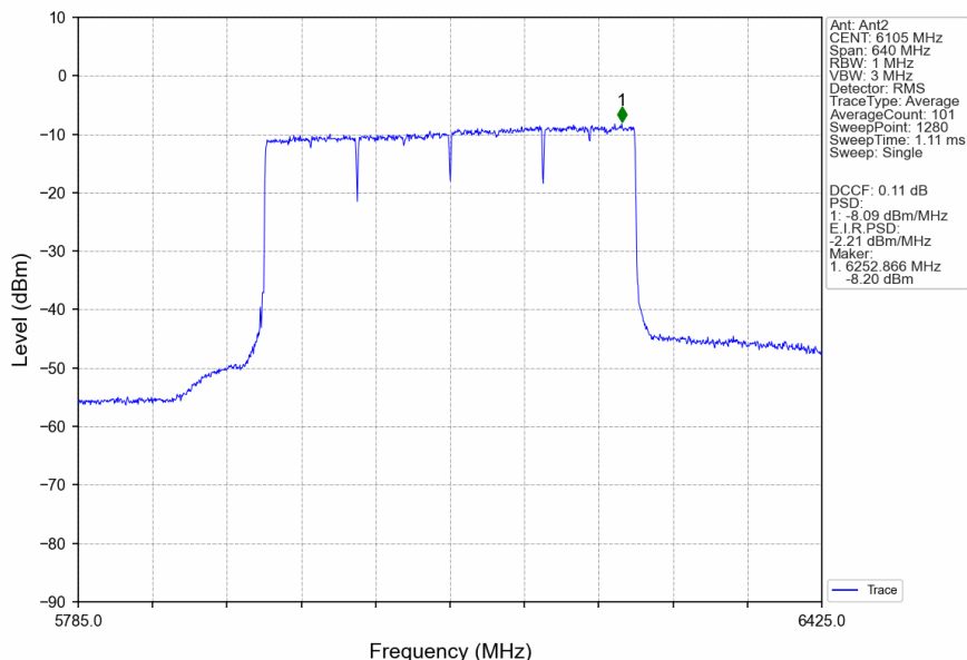
802.11be(EHT320)_LCH_6105MHz_4xRU996_Left_Ant2_NTNV
