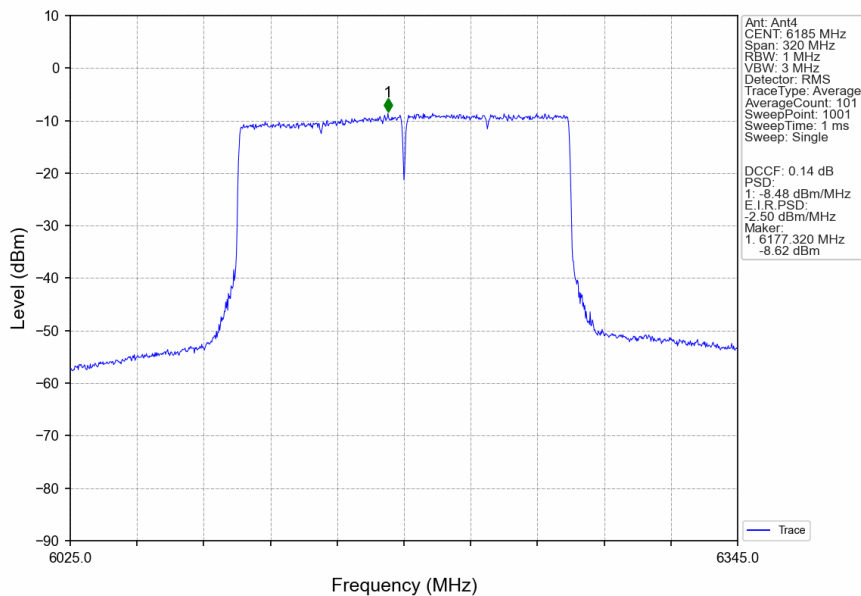
802.11be(EHT160)_MCH_6185MHz_2xRU996_Left_Ant4_NTNV
