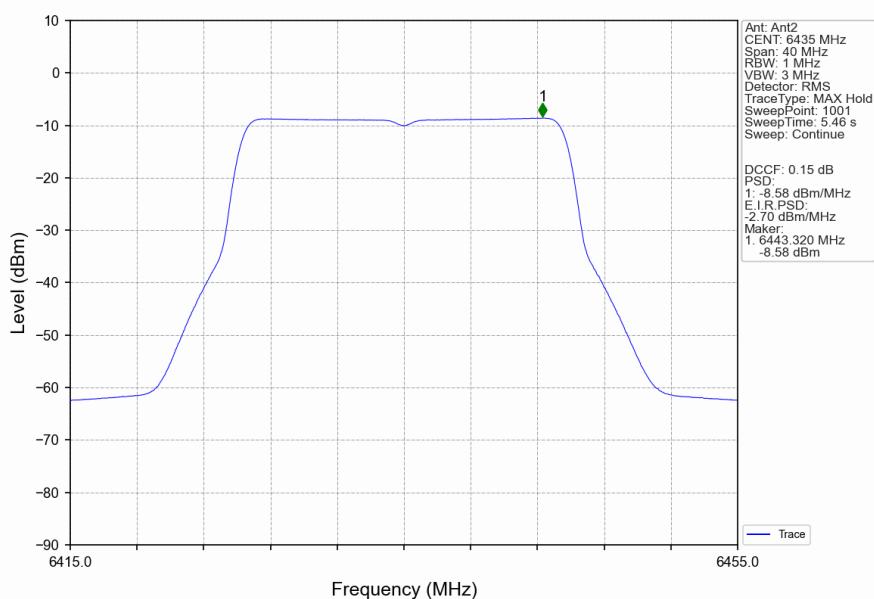
802.11be(EHT20)_LCH_6435MHz_RU242_Left_Ant2_NTNV
