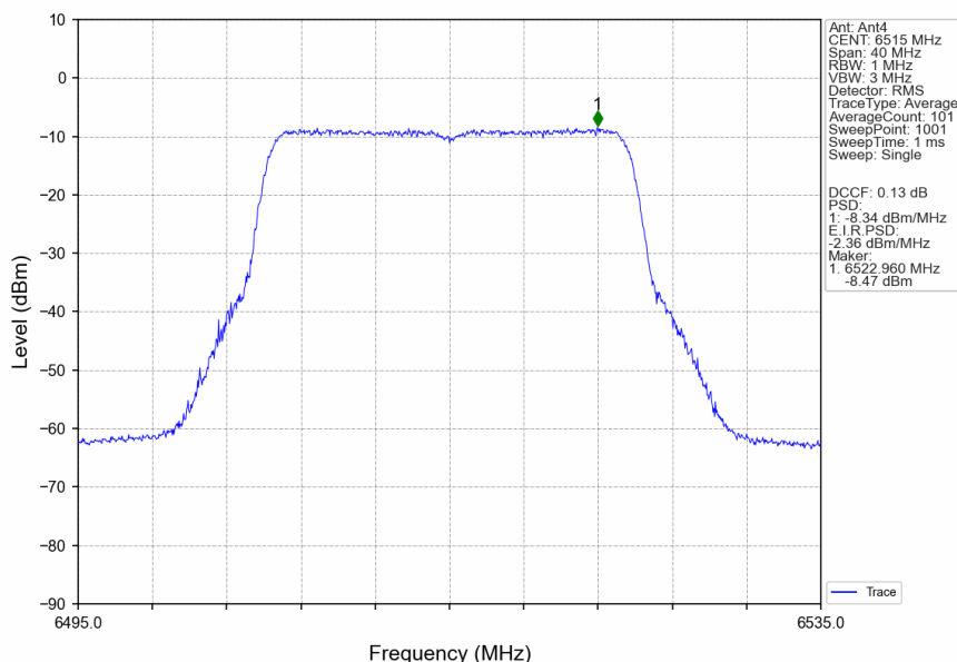
802.11be(EHT20)_HCH_6515MHz_RU242_Left_Ant4_NTNV
