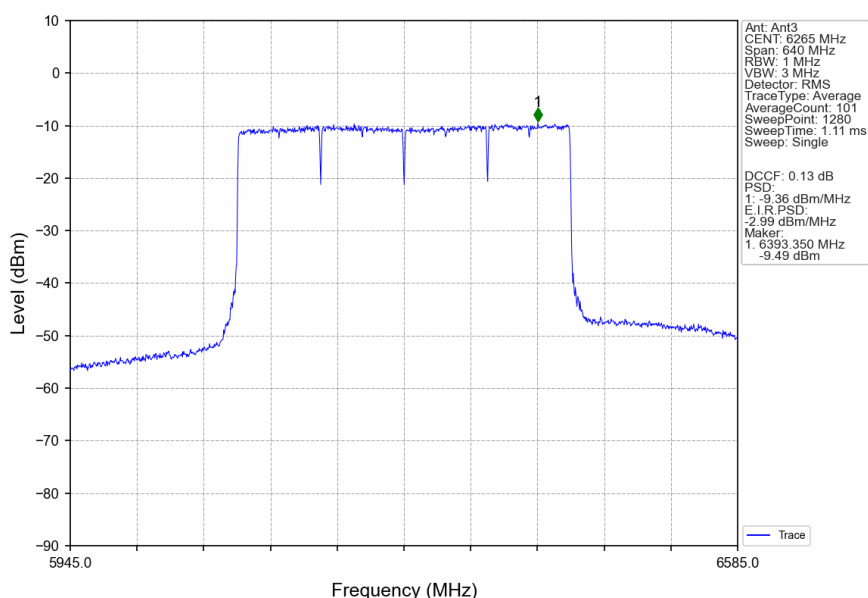
802.11be(EHT320)_HCH_6265MHz_4xRU996_Left_Ant3_NTNV
