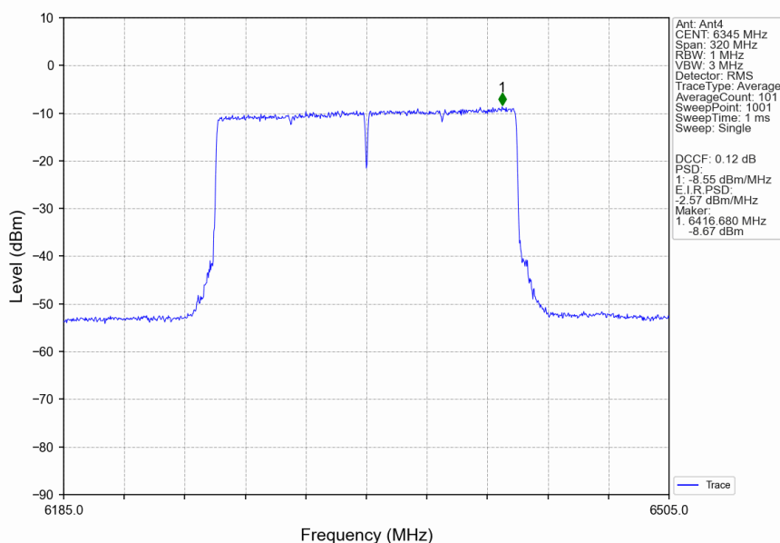
802.11be(EHT160)_HCH_6345MHz_2xRU996_Left_MIMO_NTNV
