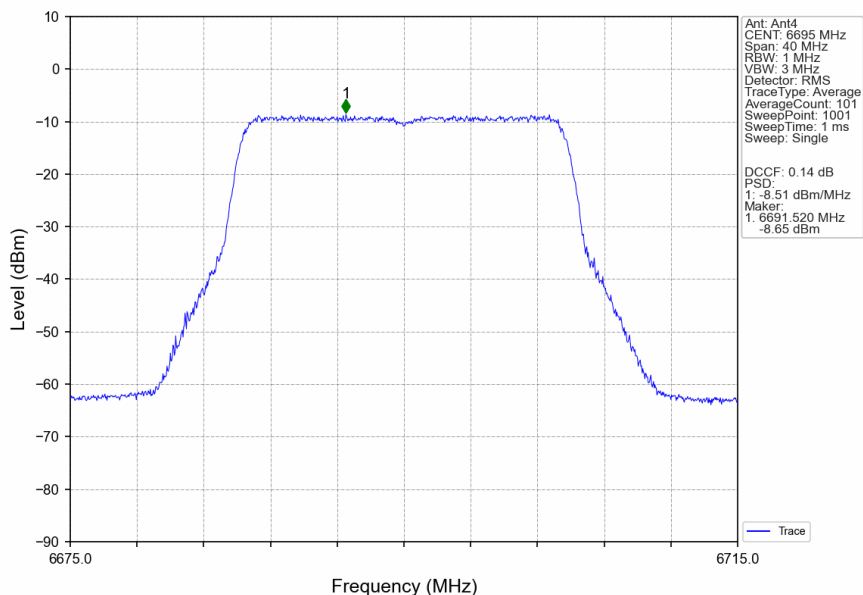
802.11be(EHT20)_MCH_6695MHz_RU242_Left_MIMO_NTNV
