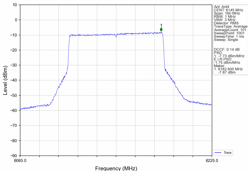
802.11be(EHT80)_MCH_6145MHz_RU996_Left_MIMO_NTNV
