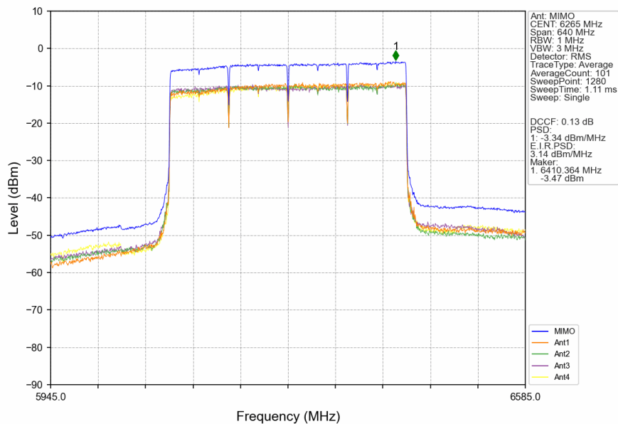
802.11be(EHT320)_HCH_6265MHz_4xRU996_Left_MIMO_NTNV
