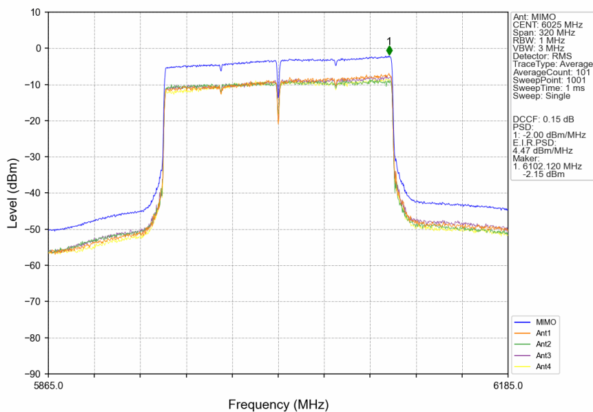
802.11be(EHT160)_LCH_6025MHz_2xRU996_Left_MIMO_NTNV
