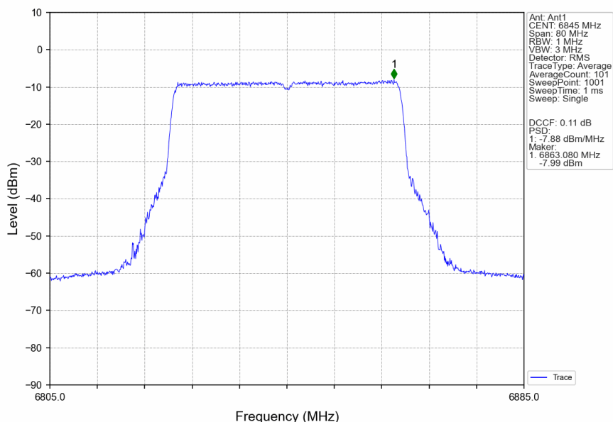
802.11be(EHT40)_HCH_6845MHz_RU484_Left_Ant1_NTNV
