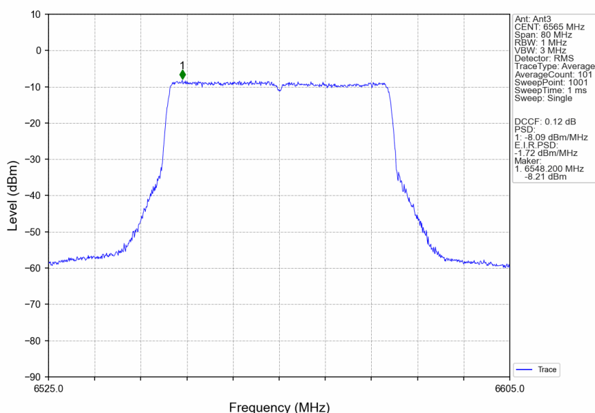
802.11be(EHT40)_LCH_6565MHz_RU484_Left_Ant3_NTNV
