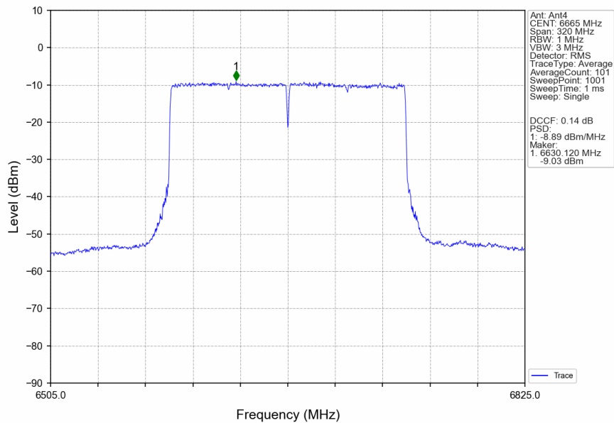
802.11be(EHT160)_MCH_6665MHz_2xRU996_Left_MIMO_NTNV
