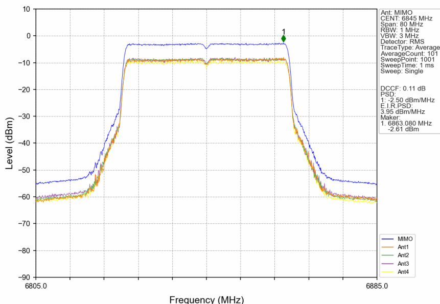
802.11be(EHT40)_HCH_6845MHz_RU484_Left_MIMO_NTNV
