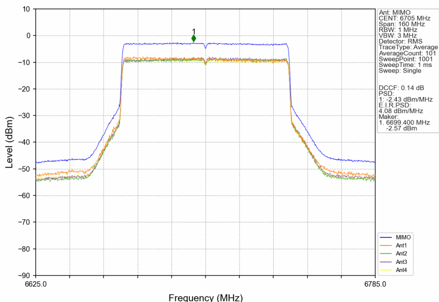
802.11be(EHT80)_MCH_6705MHz_RU996_Left_MIMO_NTNV
