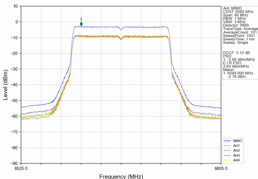
802.11be(EHT40)_LCH_6565MHz_RU484_Left_MIMO_NTNV
