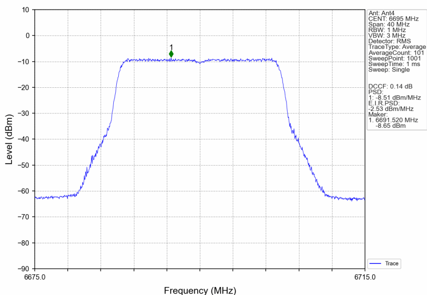
802.11be(EHT20)_MCH_6695MHz_RU242_Left_MIMO_NTNV
