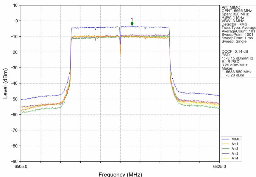
802.11be(EHT160)_MCH_6665MHz_2xRU996_Left_MIMO_NTNV
