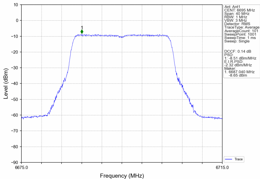
802.11be(EHT20)_MCH_6695MHz_RU242_Left_Ant1_NTNV
