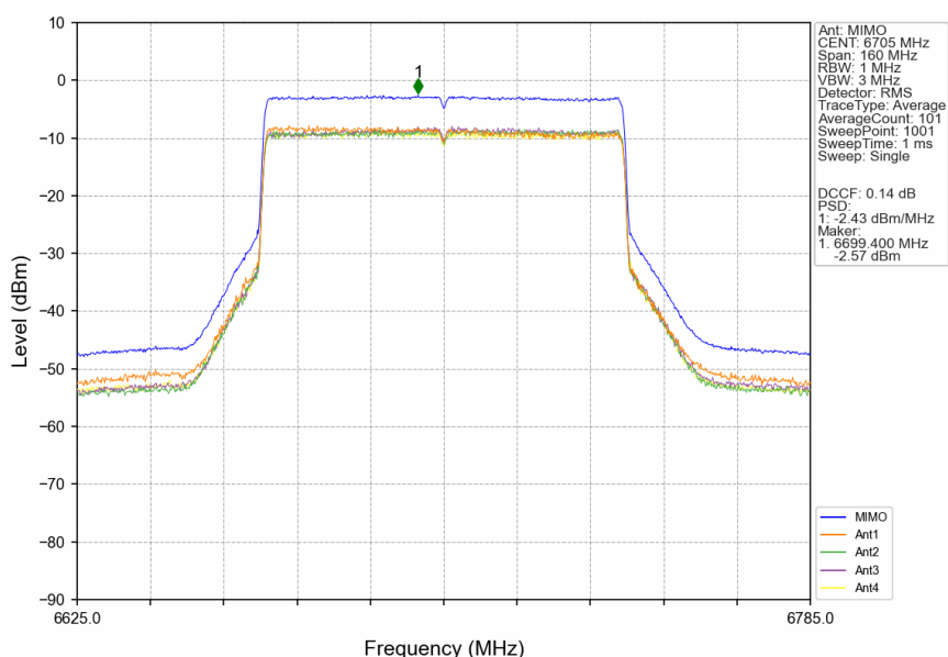
802.11be(EHT80)_MCH_6705MHz_RU996_Left_MIMO_NTNV
