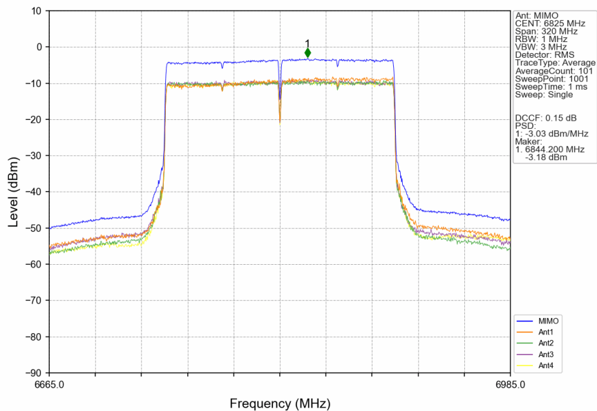
802.11be(EHT160)_HCH_6825MHz_2xRU996_Left_MIMO_NTNV
