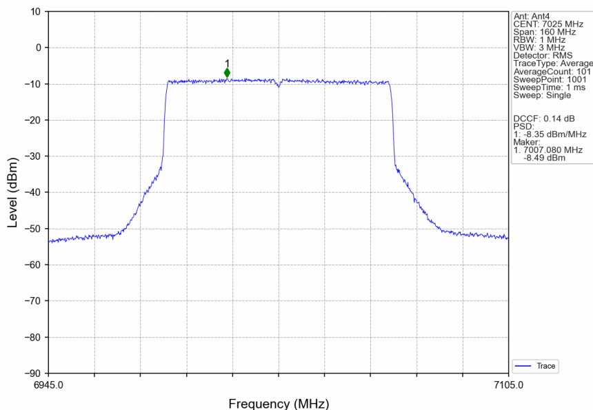
802.11be(EHT80)_HCH_7025MHz_RU996_Left_MIMO_NTNV
