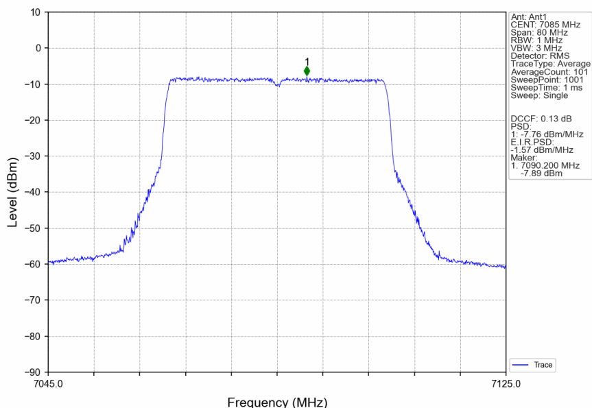
802.11be(EHT40)_HCH_7085MHz_RU484_Left_Ant1_NTNV
