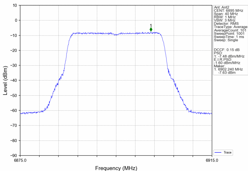
802.11be(EHT20)_LCH_6895MHz_RU242_Left_Ant2_NTNV
