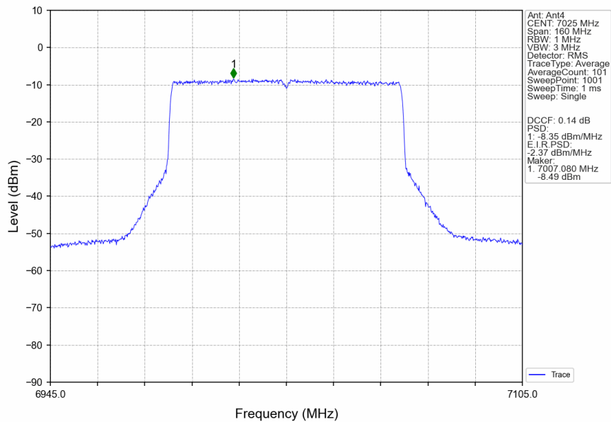
802.11be(EHT80)_HCH_7025MHz_RU996_Left_MIMO_NTNV
