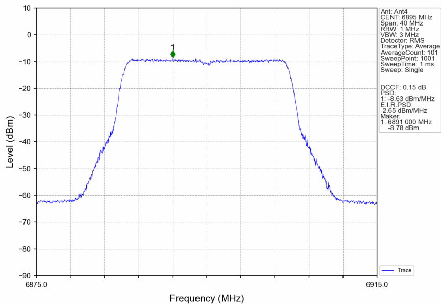
802.11be(EHT20)_LCH_6895MHz_RU242_Left_Ant4_NTNV
