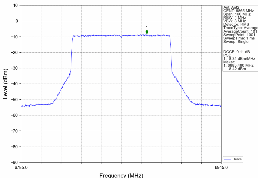
802.11be(EHT80)_HCH_6865MHz_RU996_Left_Ant2_NTNV
