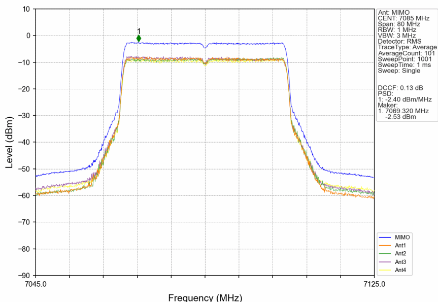
802.11be(EHT40)_HCH_7085MHz_RU484_Left_MIMO_NTNV
