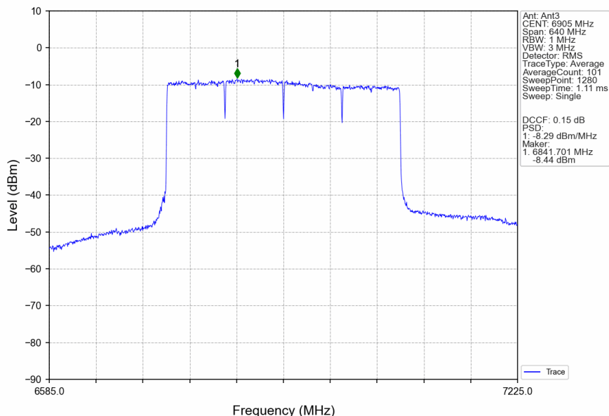
802.11be(EHT320)_HCH_6905MHz_4xRU996_Left_Ant3_NTNV
