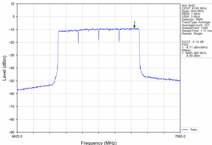
802.11be(EHT320)_LCH_6745MHz_4xRU996_Left_Ant2_NTNV
