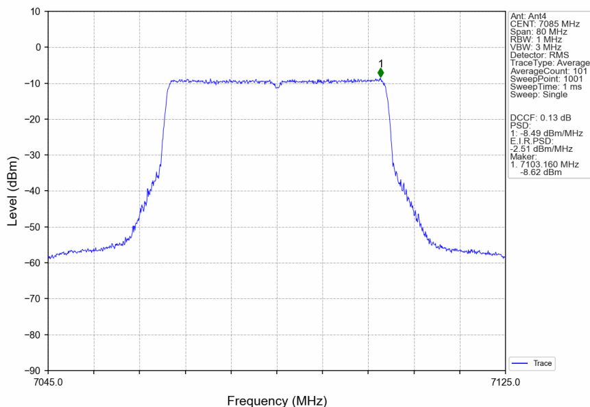
802.11be(EHT40)_HCH_7085MHz_RU484_Left_MIMO_NTNV
