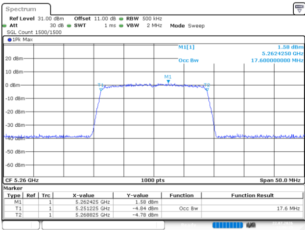
802.11ac20_5260MHz_Chain 1
