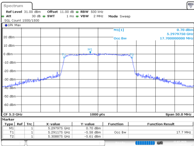
802.11ac20_5300MHz_Chain 1
