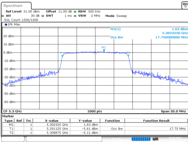
802.11ac20_5300MHz_Chain 3
