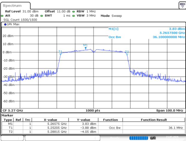
802.11ac40_5270MHz_Chain 3
