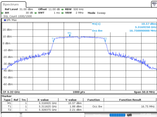
802.11a_5320MHz_Chain 3
