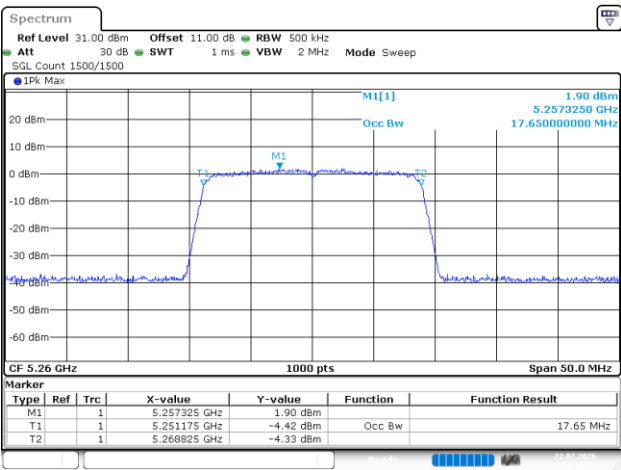
802.11ac20_5260MHz_Chain 3
