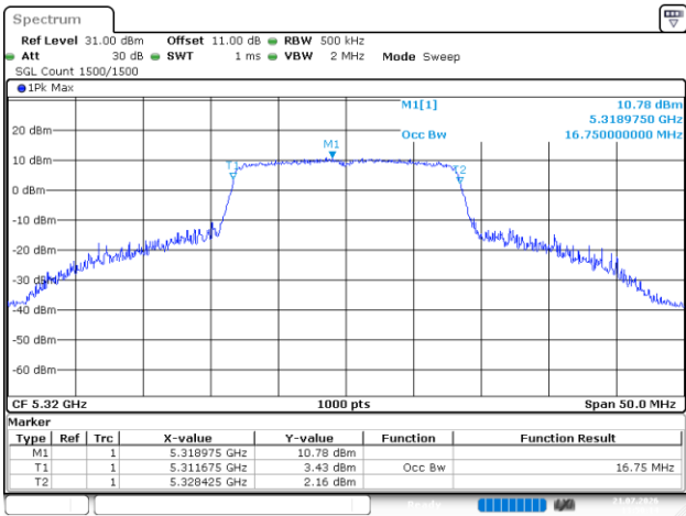
802.11a_5320MHz_Chain 4
