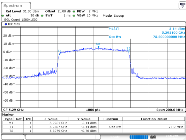
802.11ac80_5290MHz_Chain 2
