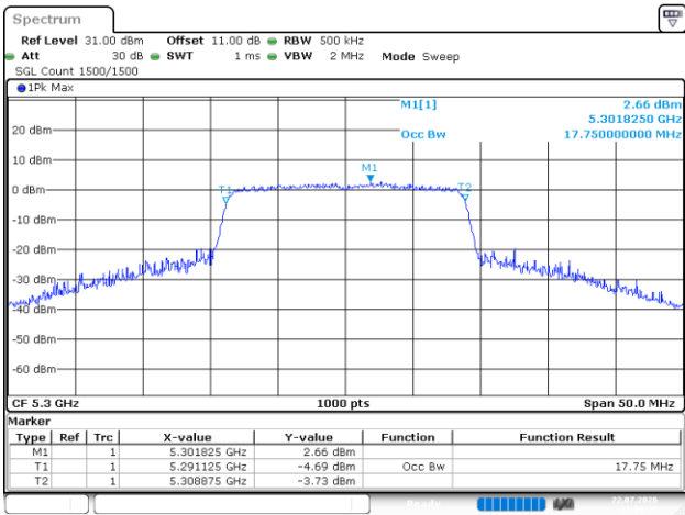
802.11ac20_5300MHz_Chain 4
