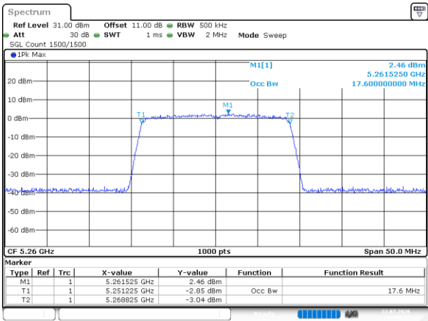
802.11ac20_5260MHz_Chain 4
