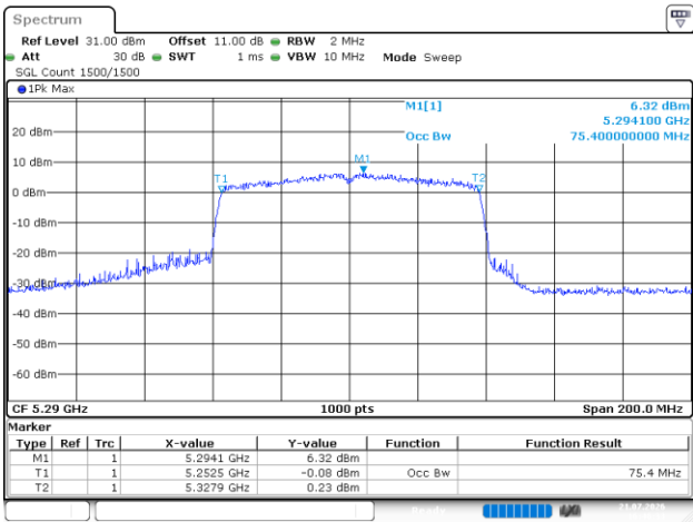
802.11ac80_5290MHz_Chain 4
