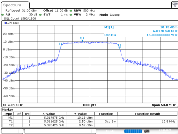
802.11a_5320MHz_Chain 1
