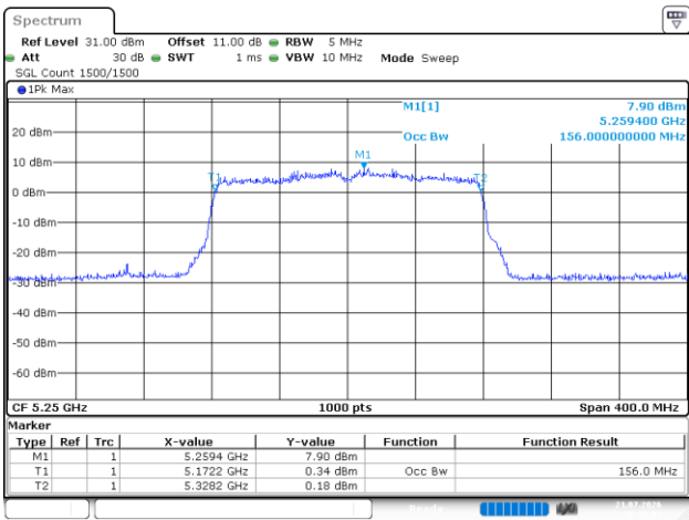
802.11ac160_5250MHz_Chain 3
