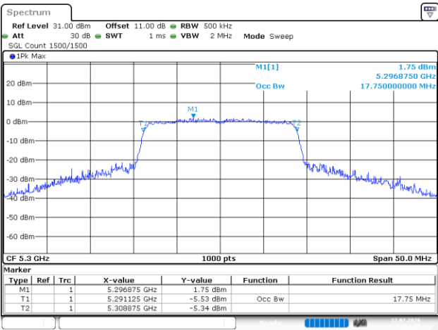
802.11ac20_5300MHz_Chain 2
