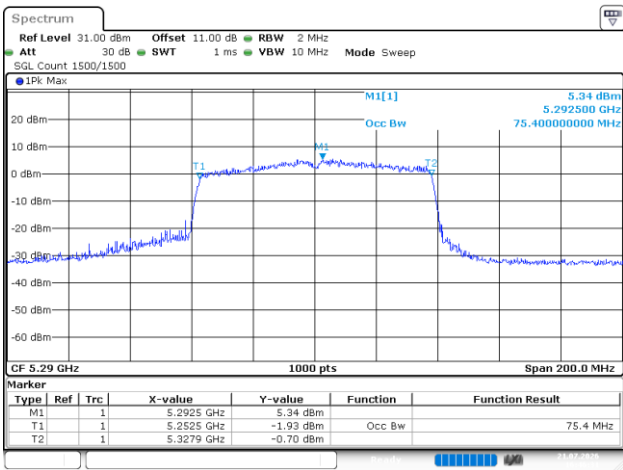
802.11ac80_5290MHz_Chain 3
