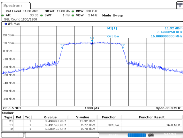
802.11a_5500MHz_Chain 3
