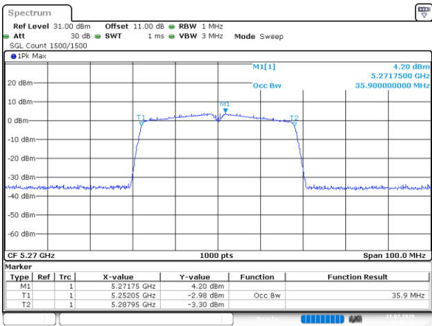
802.11ac40_5270MHz_Chain 0
