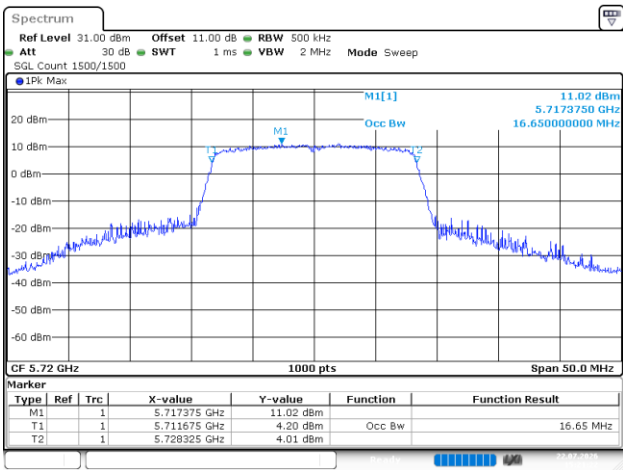
802.11a_5720MHz_Chain 2
