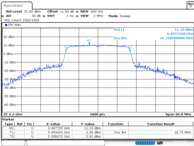
802.11a_5500MHz_Chain 4
