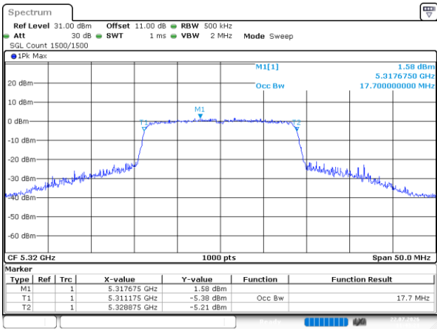
802.11ac20_5320MHz_Chain 3
