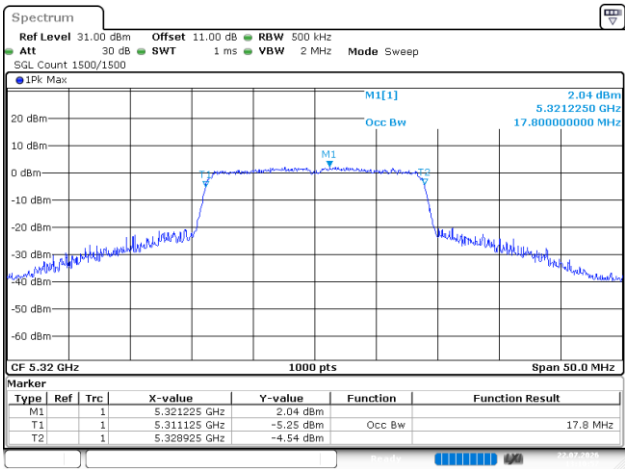
802.11ac20_5320MHz_Chain 4
