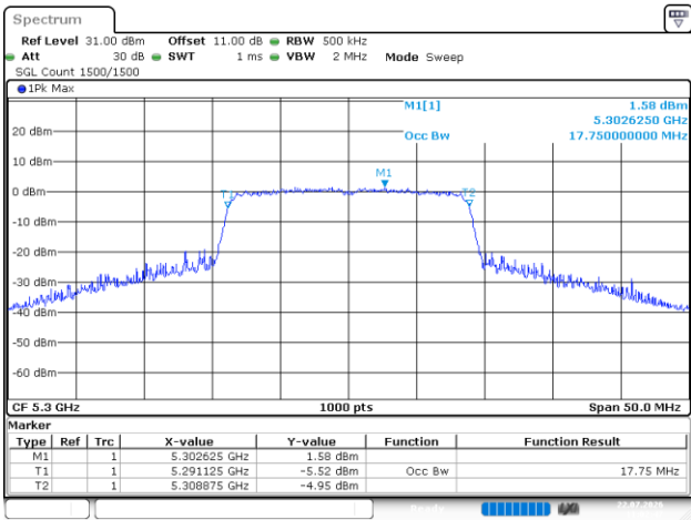
802.11ac20_5300MHz_Chain 0
