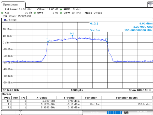
802.11ac160_5250MHz_Chain 4
