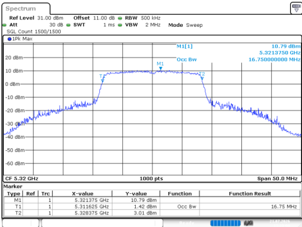
802.11a_5320MHz_Chain 2
