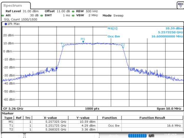
802.11a_5260MHz_Chain 4
