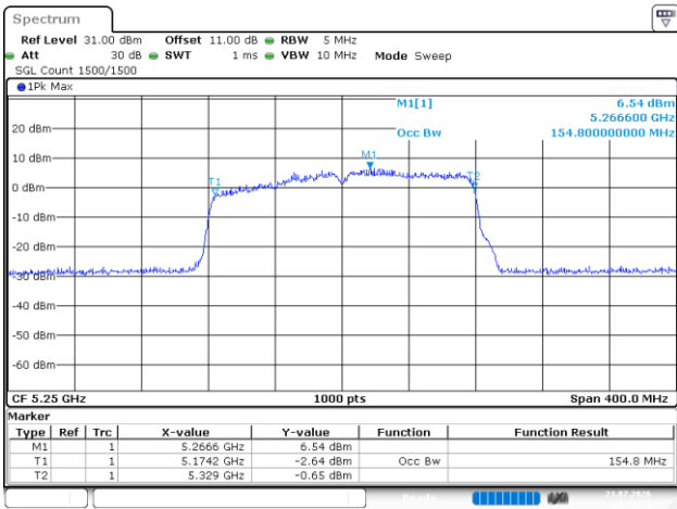
802.11ac160_5250MHz_Chain 2
