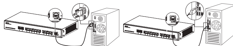
Connexion au port de console (USB)
