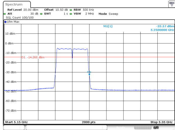
802.11ac40_5230MHz
