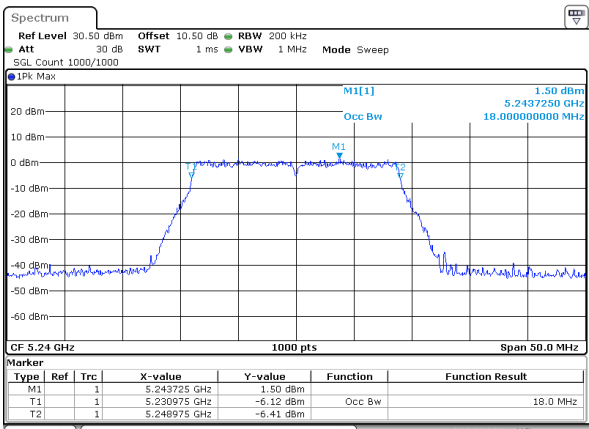
802.11ac20_5240MHz
