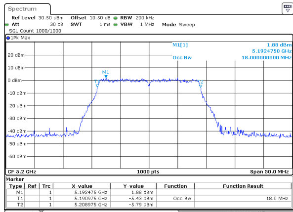
802.11ac20_5200MHz
