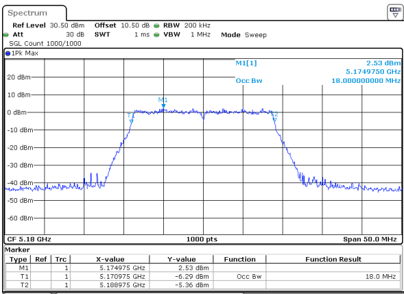
802.11ac20_5180MHz
