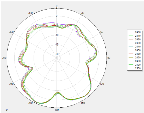
2.4G phi=0deg
