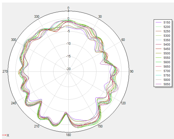
5G phi=0deg
