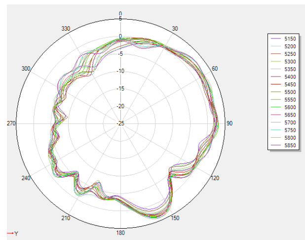
5G phi=90deg
