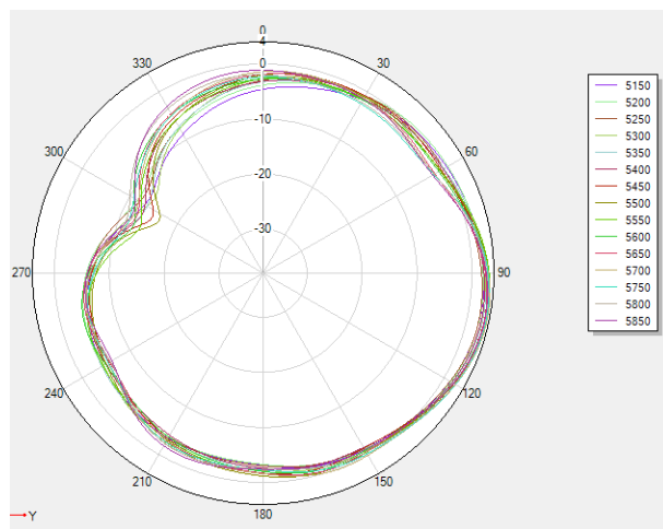
5G theta=90deg
