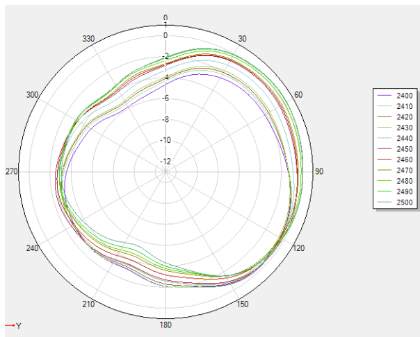
2.4G theta=90deg
