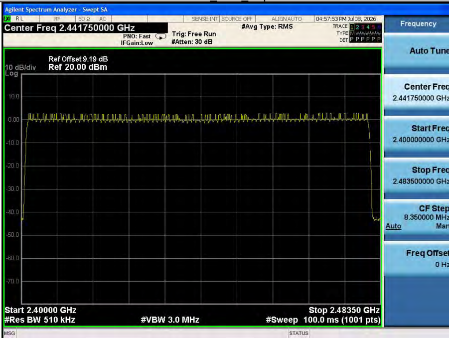
3DH5_Ant1_Hop
