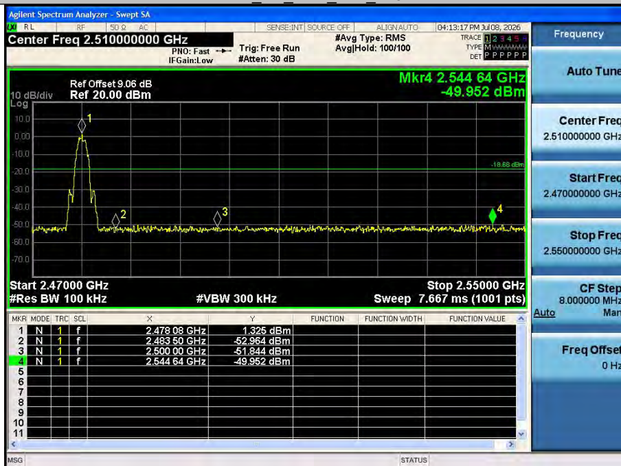
BLE 2M Ant1 High 2478
