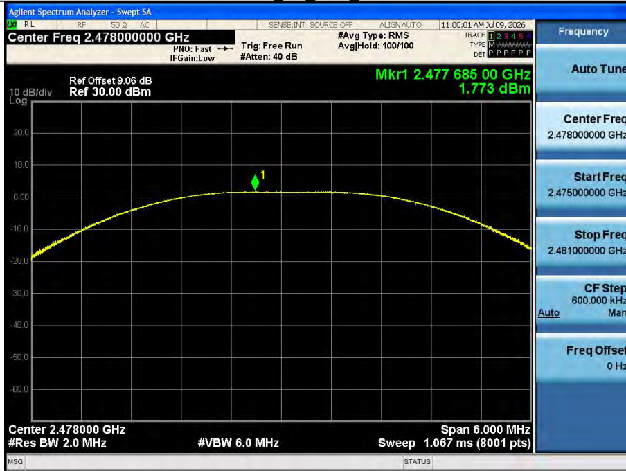
BLE 2M Ant1_2478
