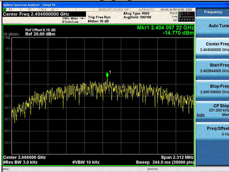
BLE 2M Ant1_2404
