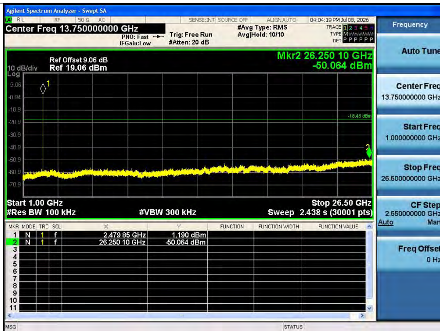
BLE_1M_Ant1_2480_1000~26500
