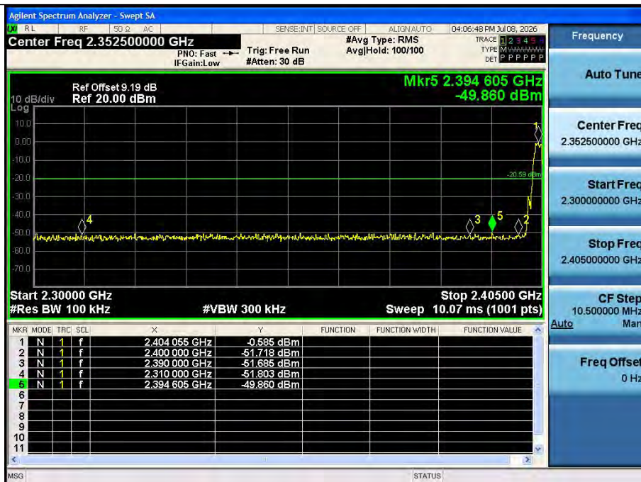
BLE 2M Ant1 Low 2404
