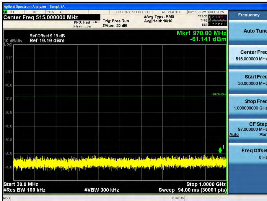
BLE 2M Ant1 2404 30~1000
