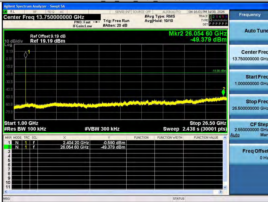
BLE 2M Ant1 2404 1000~26500
