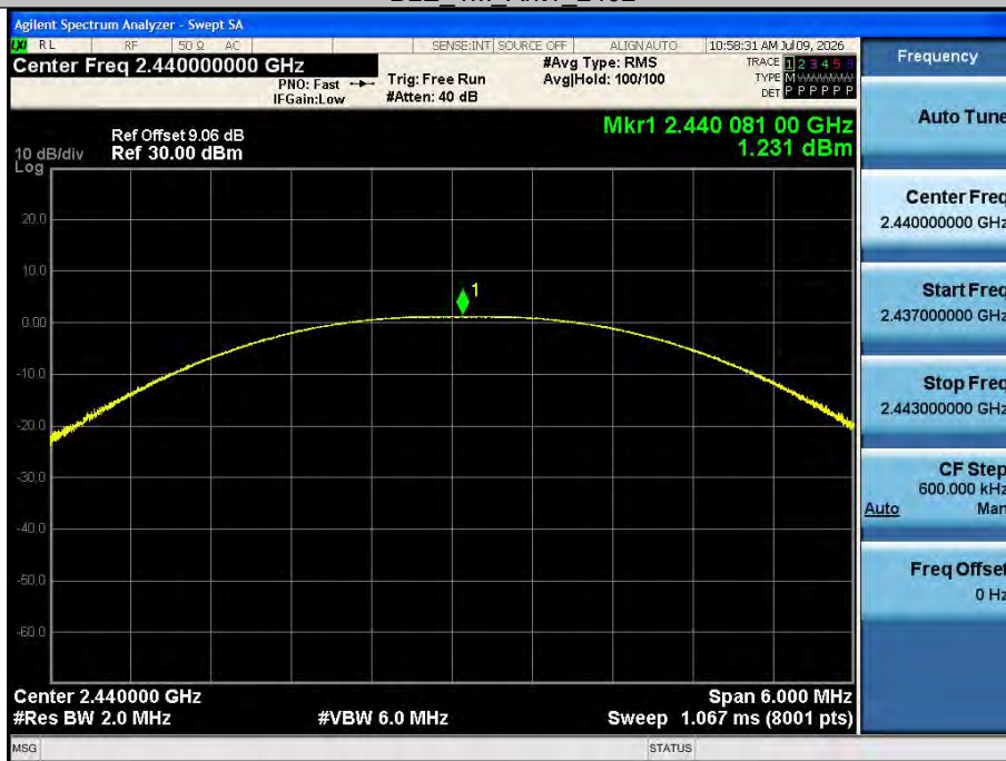
BLE_1M Ant1 2440
