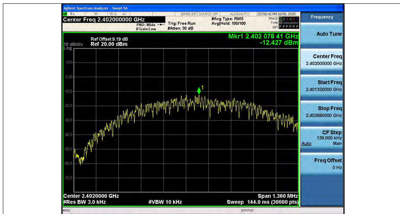
BLE_1M Ant1 2402
