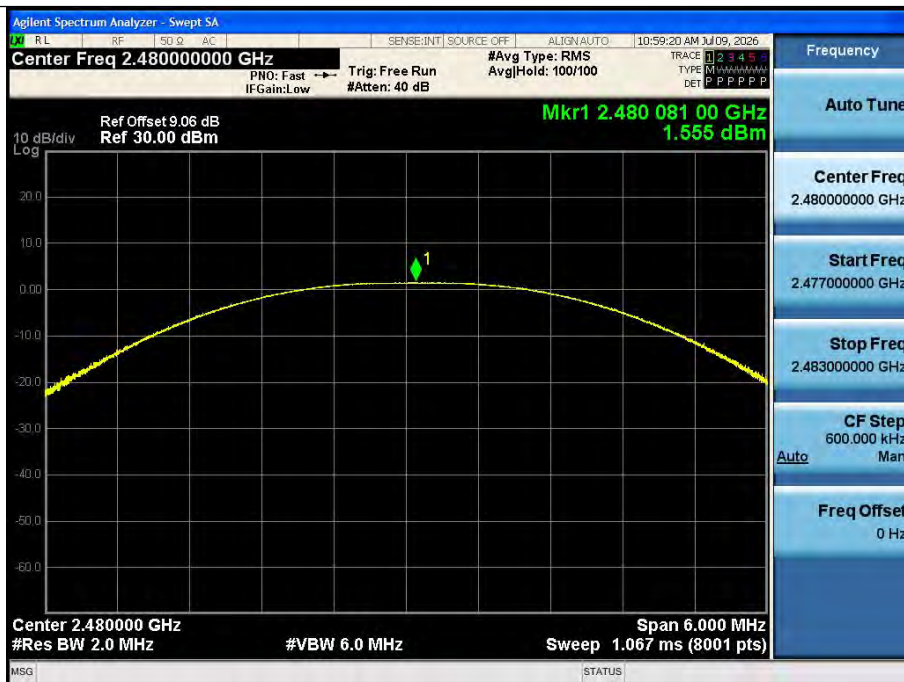
BLE 1M Ant1_2480
