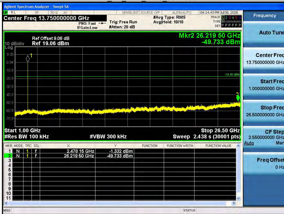
BLE_2M_Ant1_2478_1000~26500
