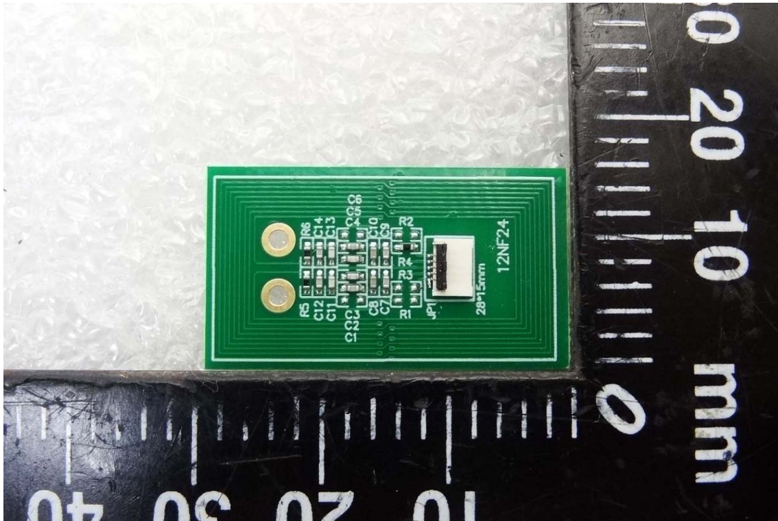
EUT 14 Antenna
