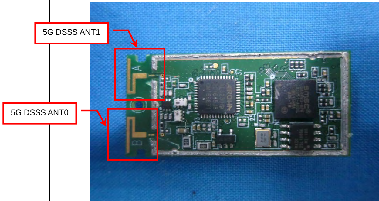
EUT Photo (18)
