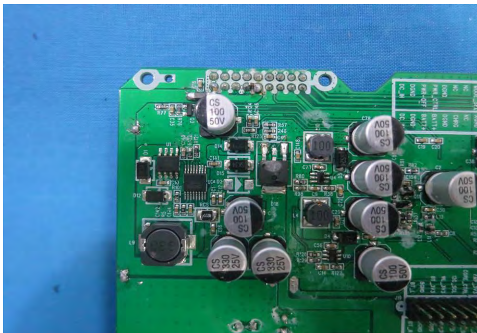
EUT Photo (12)
