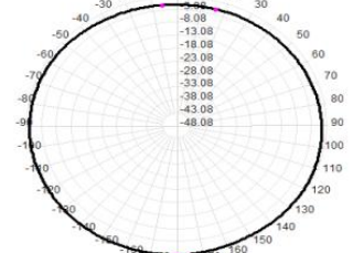
2400.0MHz Total(H), Max= 1.75dBi
