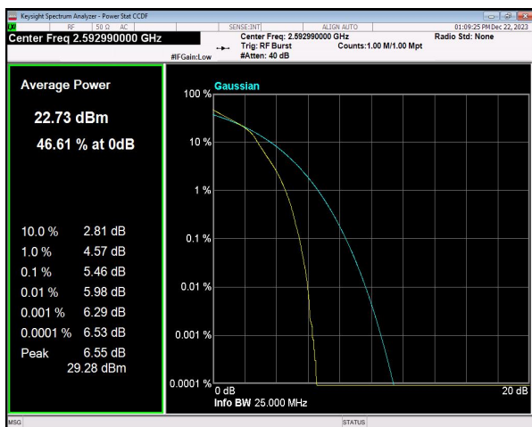
n41 SCS=30kHz DFT_16QAM BW=20MHz Channel=518598 RB=50@0
