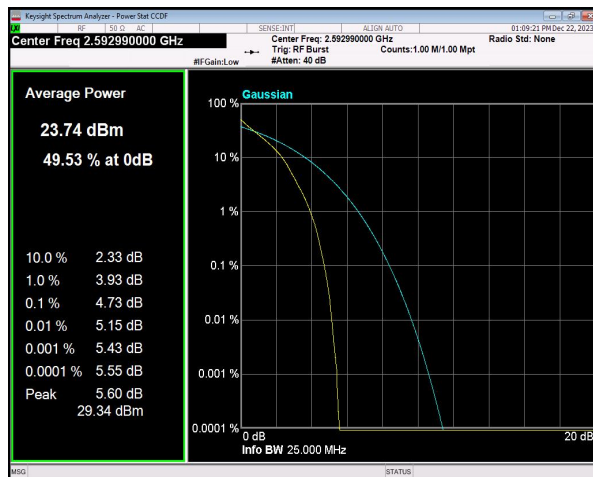
n41 SCS=30kHz DFT_QPSK BW=20MHz Channel=518598 RB=50@0
