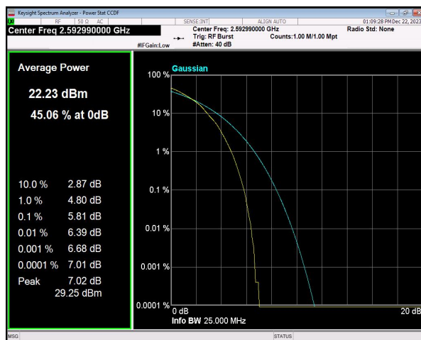
n41 SCS=30kHz DFT_64QAM BW=20MHz Channel=518598 RB=50@0
