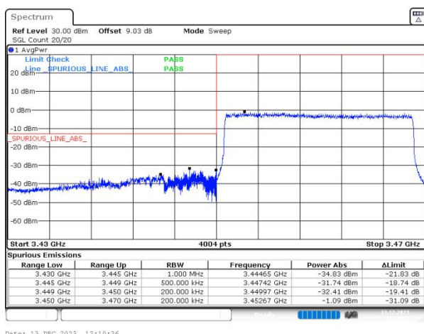
n77(3450-3550) SCS=30kHz DFT_QPSK BW=20MHz LowChannel=630668 RB=50@0
