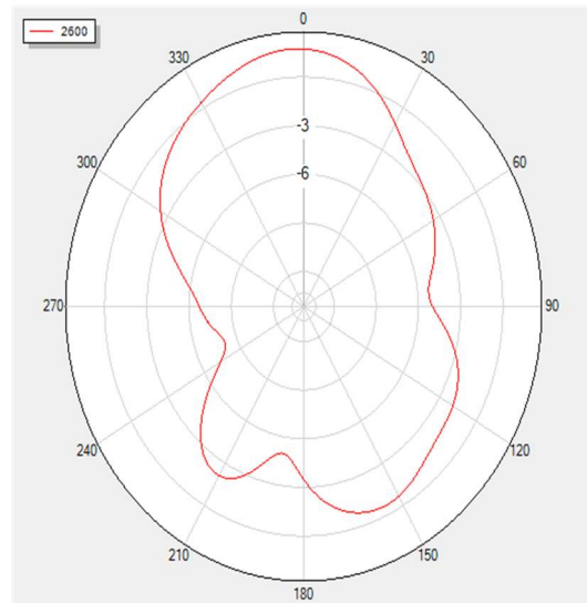
V Phi=0
