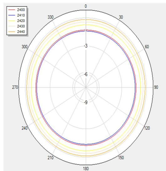
H Theta=0
