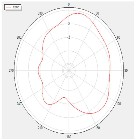
V Phi=90
