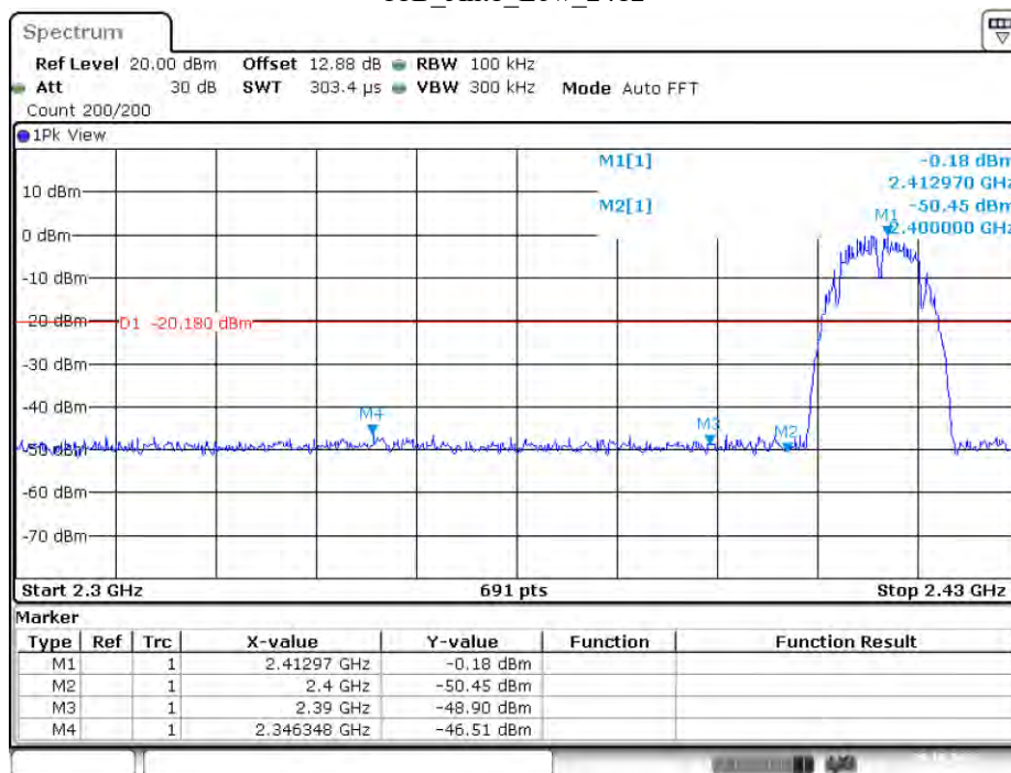
11B_Ant1_Low_2412
