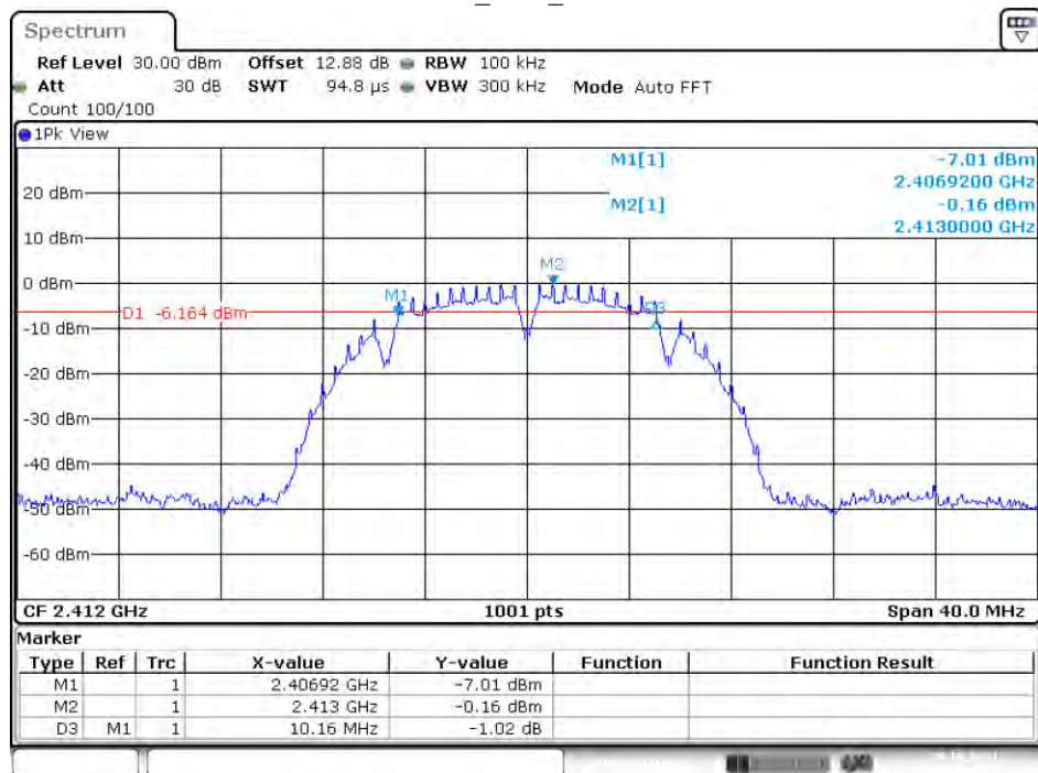
11B_Ant1_2412
