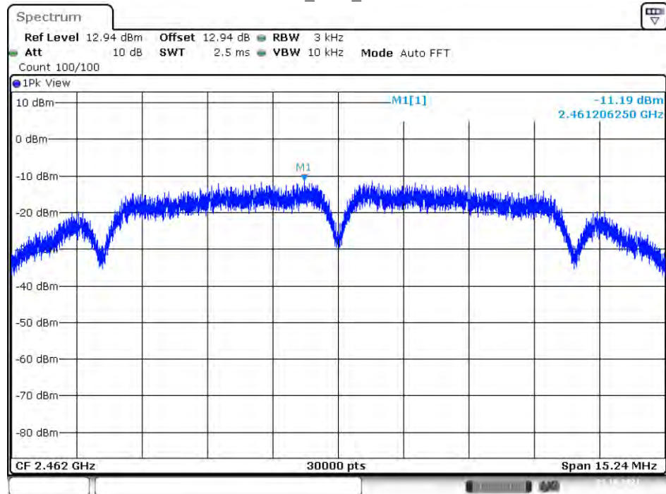
11B_Ant1_2462
