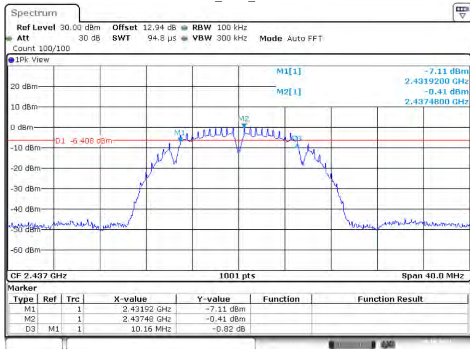
11B_Ant1_2437
