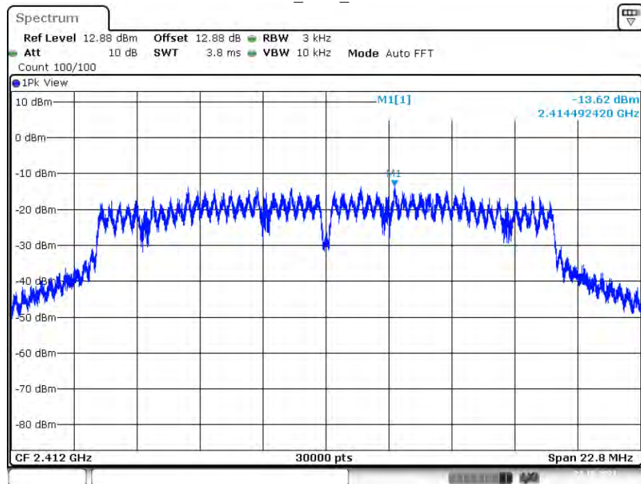
11G_Ant1_2412
