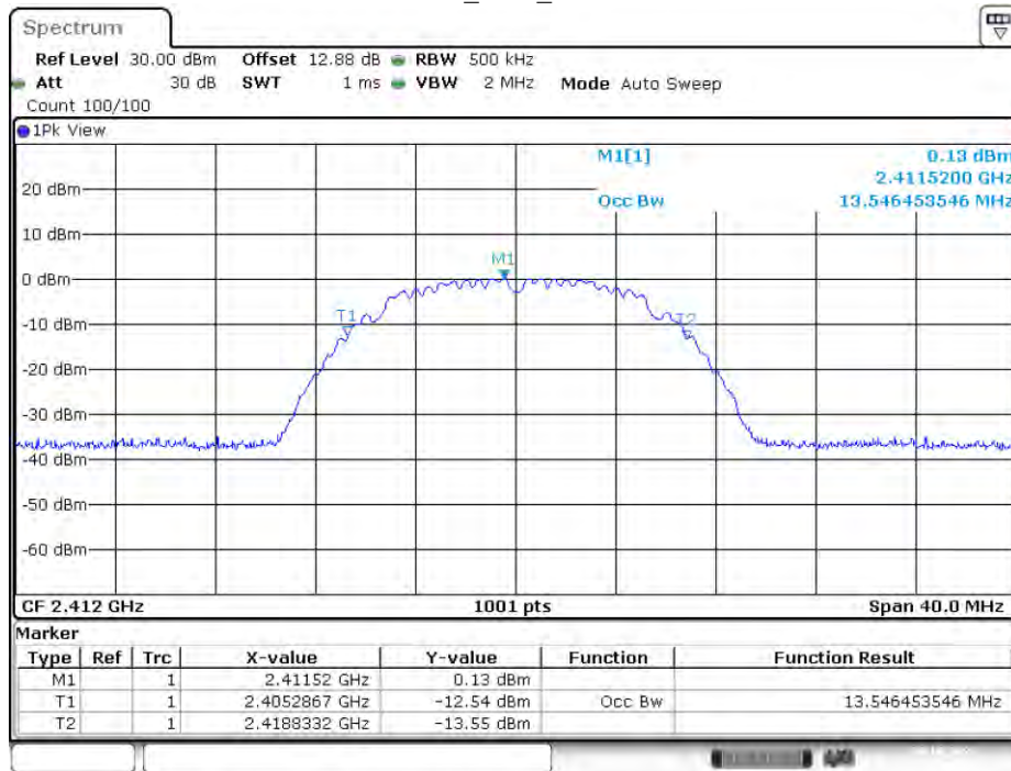
11B_Ant1_2412
