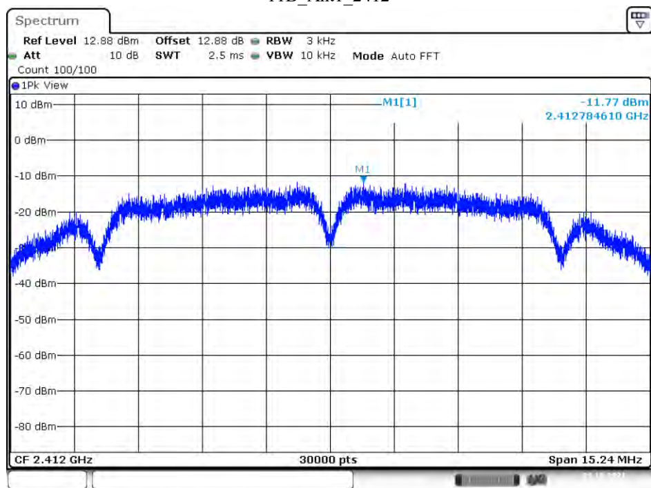
11B_Ant1_2412
