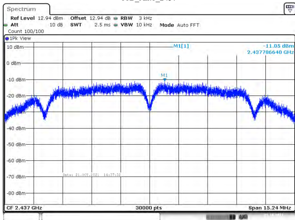
11B_Ant1_2437
