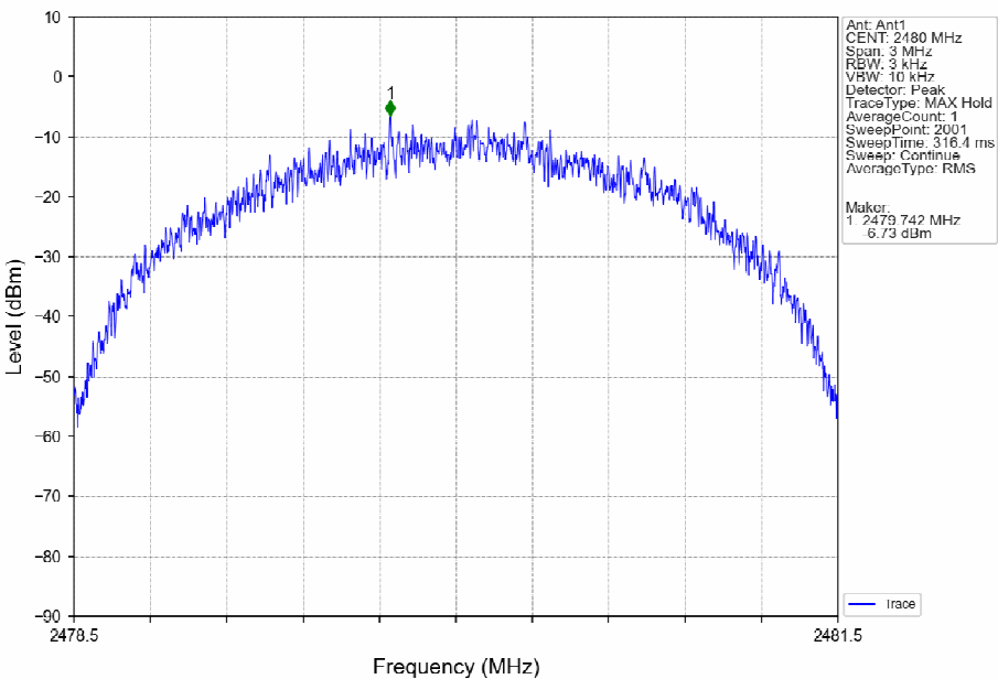
2M_HCH_2480MHz_Ant1_NTNV
