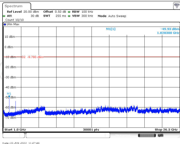
BW500K_Ant1_914.2_1000~26500
