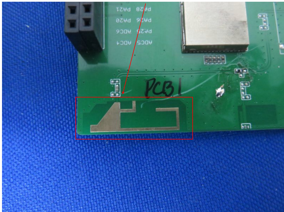
ANT A
