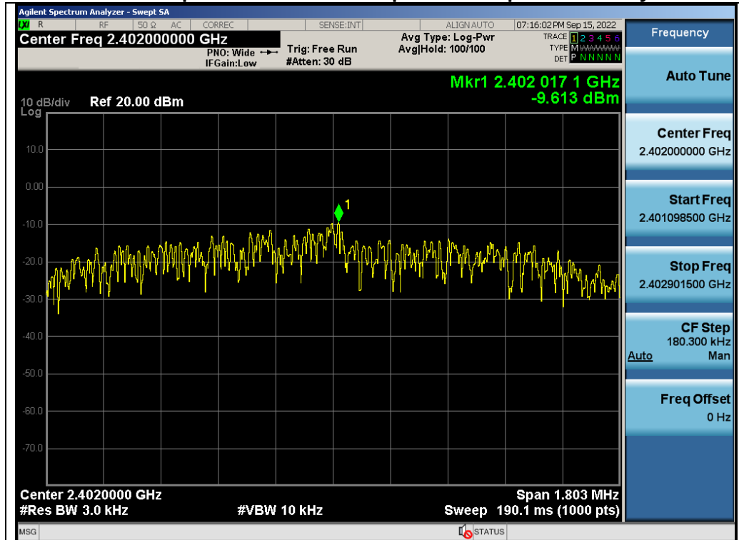
Test_Graph_LE2M_ANT1_2402_2Mbps_PSD
