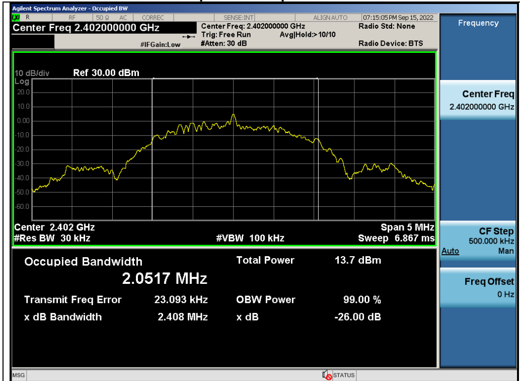
Test_Graph_LE2M_ANT1_2402_2Mbps_OBW
