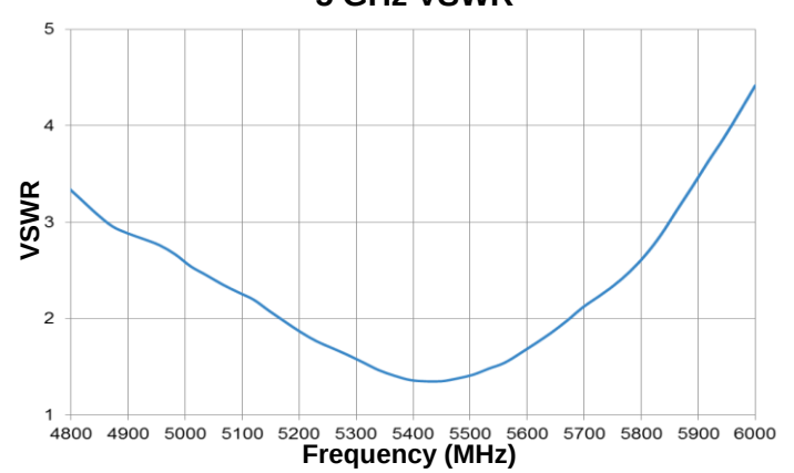
5 GHz VSWR
