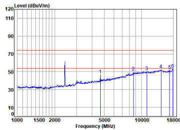
11ax_20M_TX_CH_01_Horizontal
