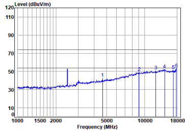
11b_TX_CH_11_Horizontal
