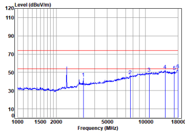
11b_TX_CH_01_Horizontal
