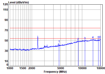
11ax_40M_TX_CH_03_Horizontal
