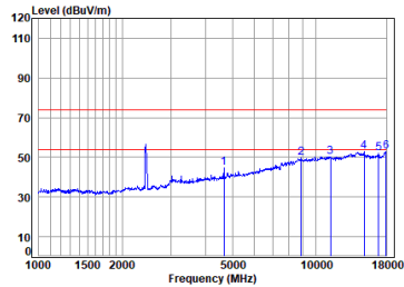
11ax_40M_TX_CH_06_Horizontal
