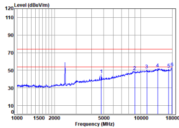
11ax_20M_TX_CH_06_Horizontal
