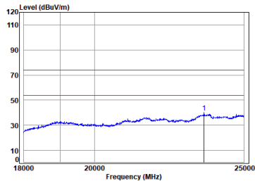
11n_40M_TX_CH_03_Horizontal
