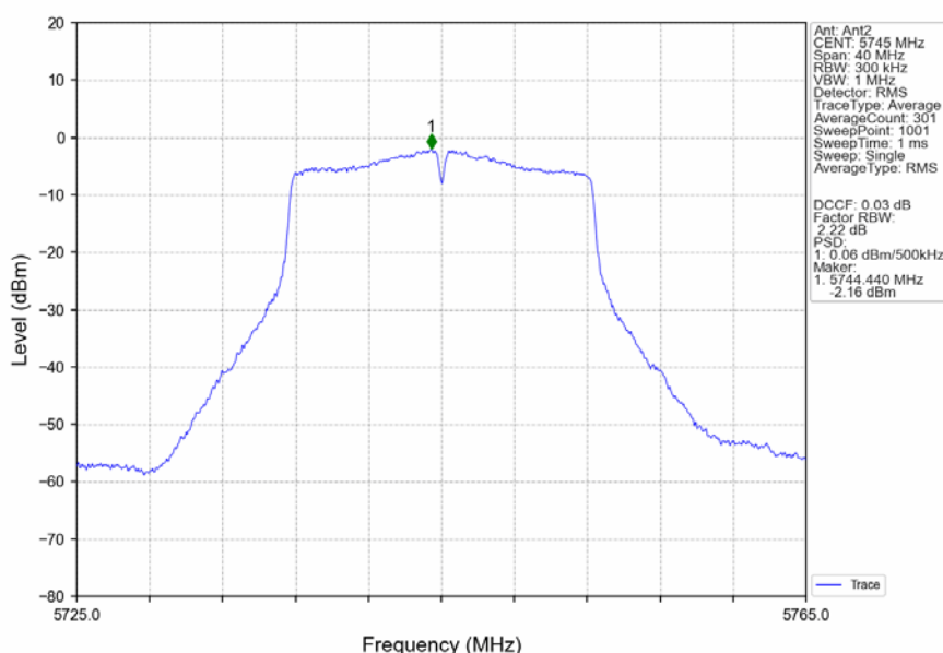
802.11a_LCH_5745MHz_Ant2_NTNV
