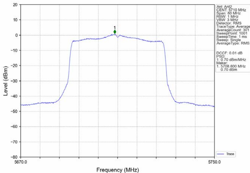
802.11ax(HEW40)_HCH_5710MHz_RU484_Left_Ant2_NTNV
