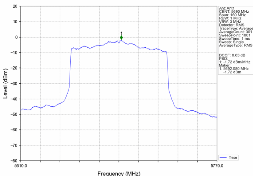
802.11ax(HEW80)_HCH_5690MHz_RU996_Left_Ant1_NTNV
