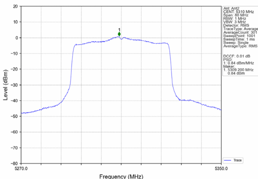
802.11ax(HEW40)_HCH_5310MHz_RU484_Left_Ant2_NTNV
