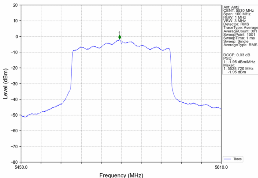
802.11ax(HEW80)_LCH_5530MHz_RU996_Left_MIMO_NTNV
