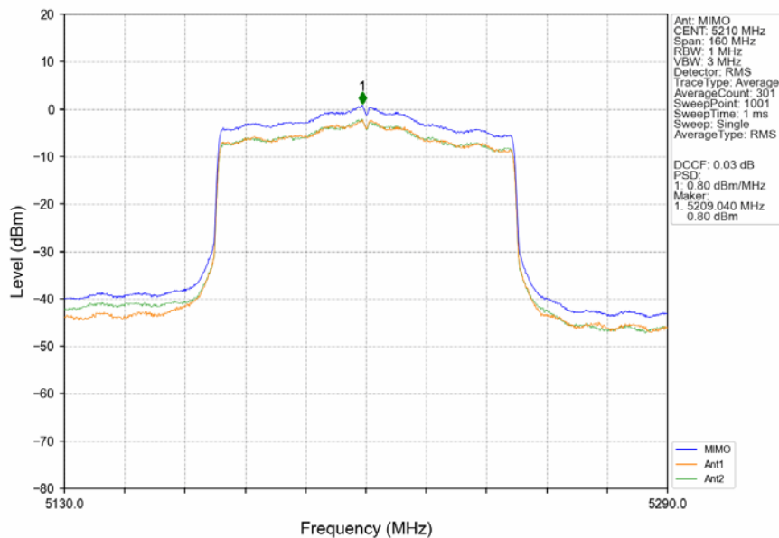
802.11ax(HEW80)_MCH_5210MHz_RU996_Left_MIMO_NTNV
