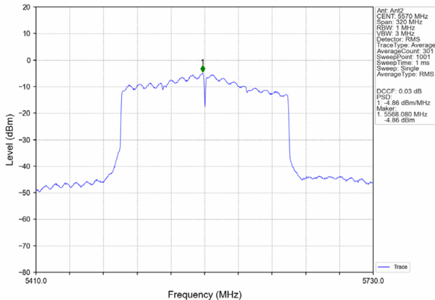
802.11ax(HEW160)_MCH_5570MHz_2xRU996_Left_Ant2_NTNV
