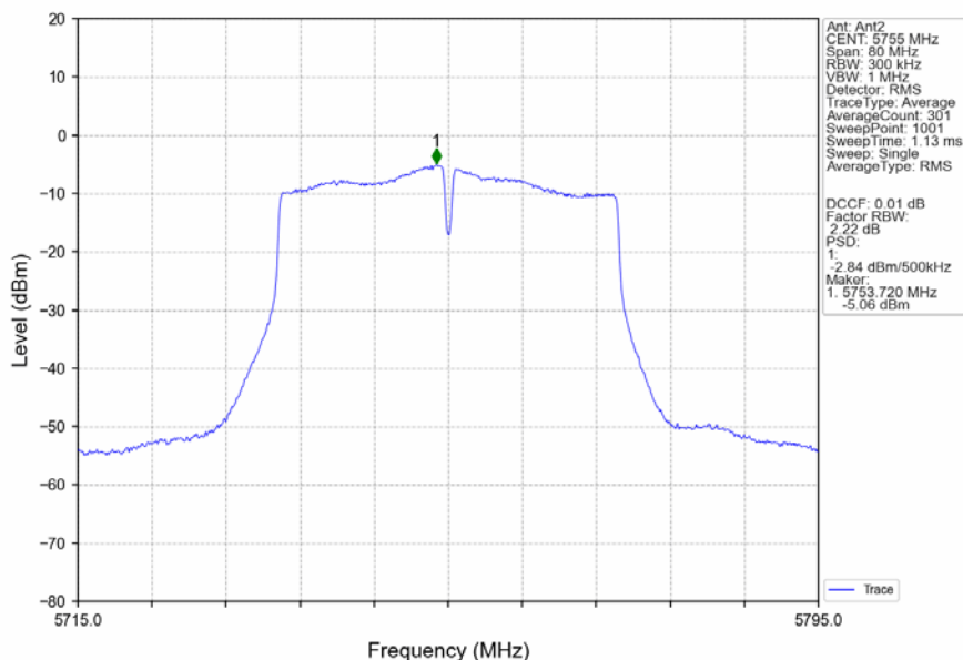
802.11ac(VHT40)_LCH_5755MHz_MIMO_NTNV
