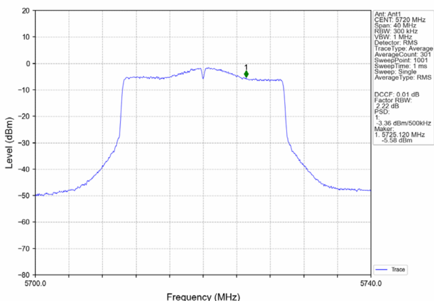
802.11ax(HEW20)_HCH_5720MHz_RU242_Left_Ant1_NTNV
