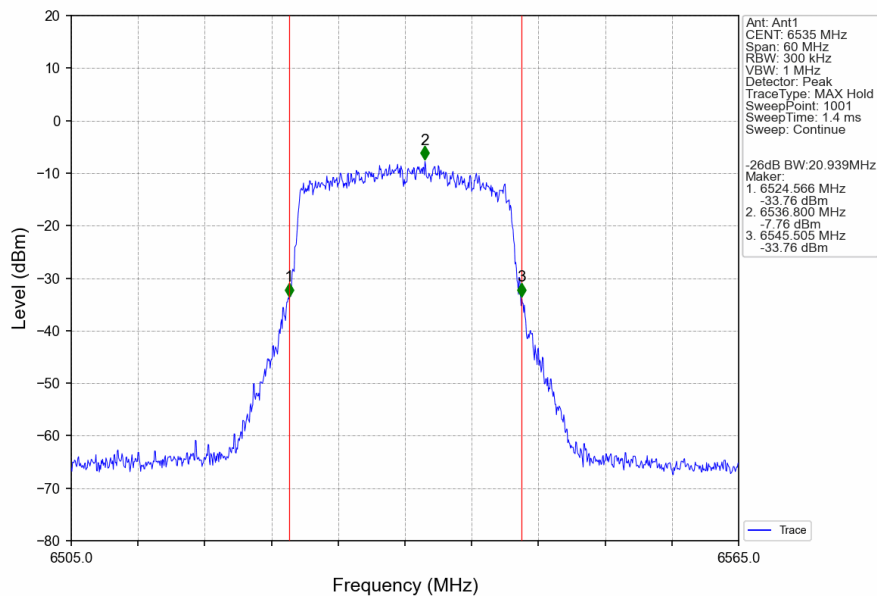
802.11ax(HEW20)_LCH_6535MHz_RU242_Left_Ant1_NTNV
