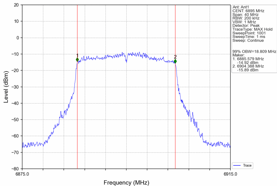
802.11ax(HEW20)_LCH_6895MHz_RU242_Left_Ant1_NTNV
