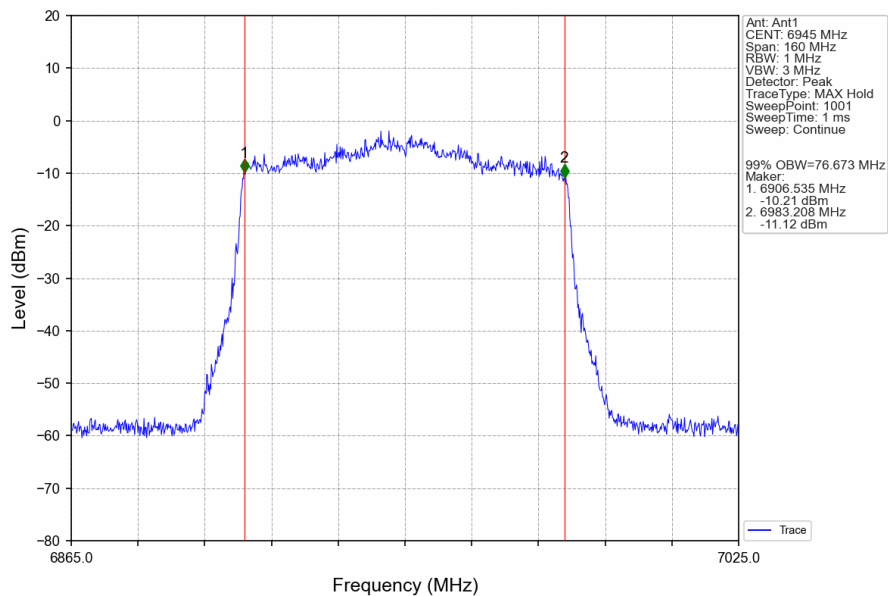
802.11ax(HEW80)_LCH_6945MHz_RU996_Left_Ant1_NTNV
