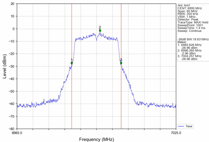
802.11a_MCH_6995MHz_Ant1_NTNV
