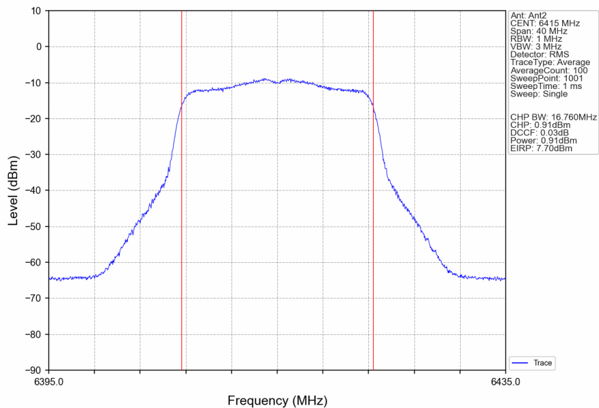
802.11a_HCH_6415MHz_Ant2_NTNV
