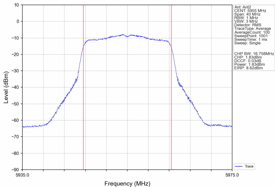
802.11a_LCH_5955MHz_Ant2_NTNV
