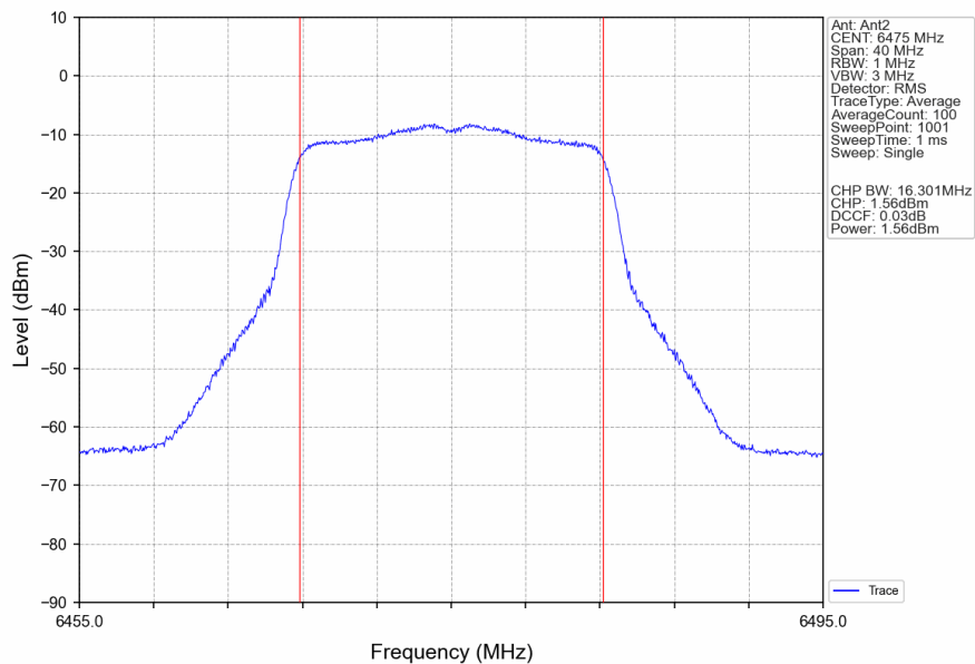
802.11a_MCH_6475MHz_Ant2_NTNV
