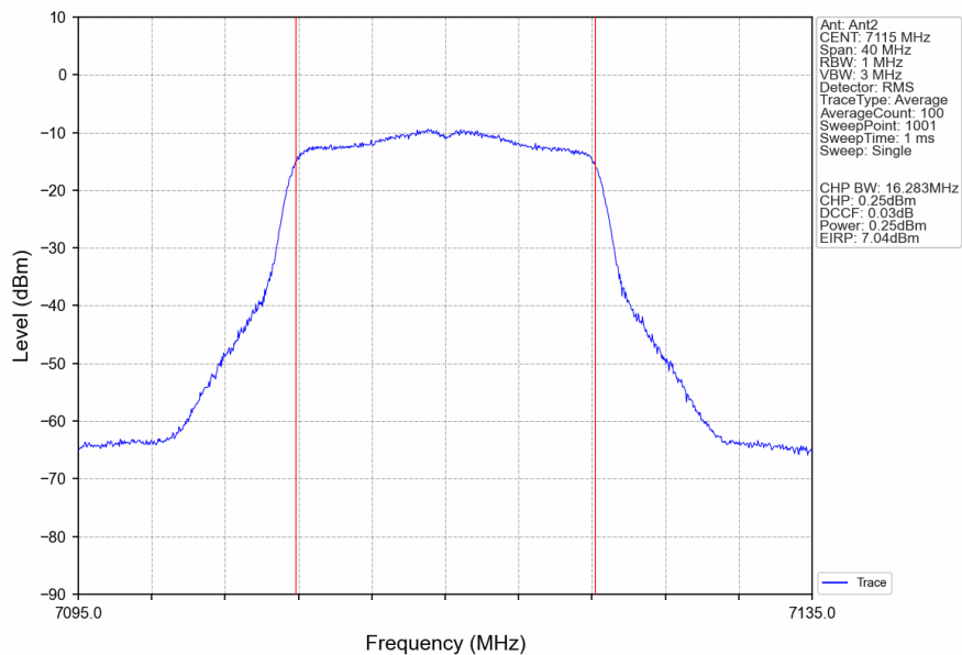
802.11a_HCH_7115MHz_Ant2_NTNV
