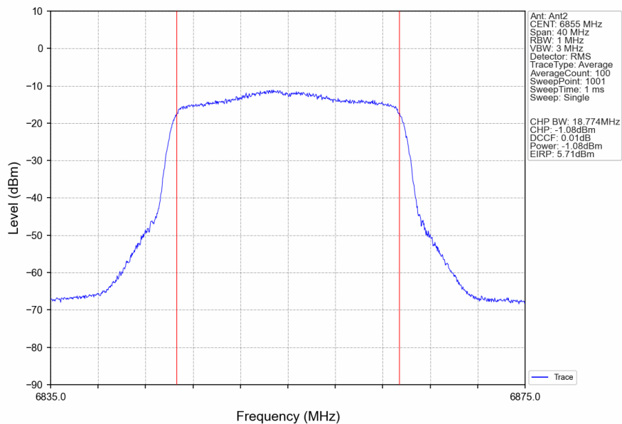
802.11ax(HEW20)_HCH_6855MHz_RU242_Left_Ant2_NTNV
