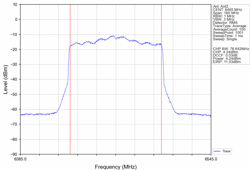
802.11ax(HEW80)_LCH_6465MHz_RU996_Left_Ant2_NTNV
