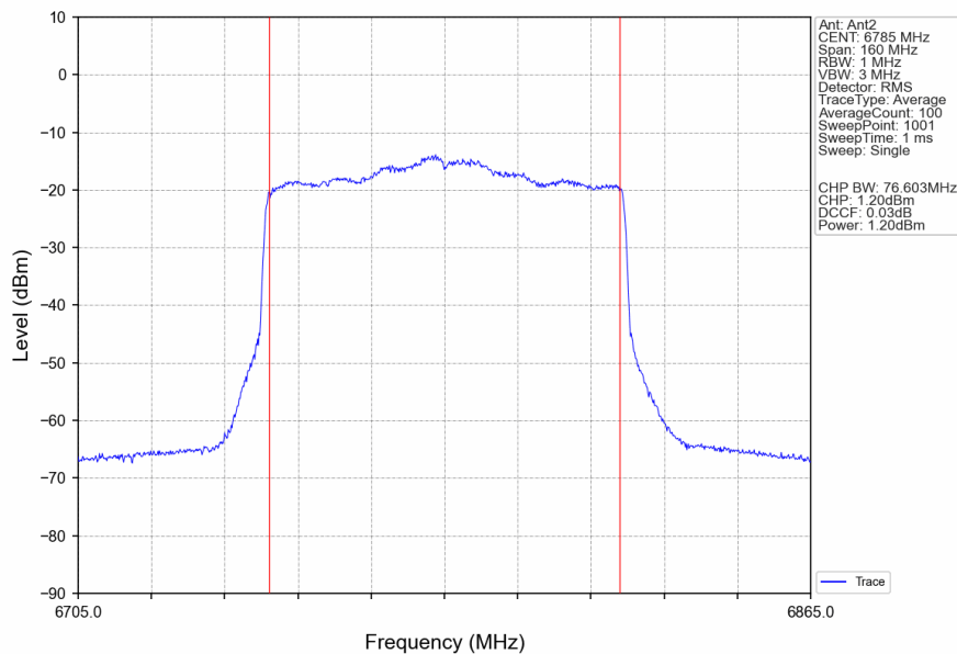
802.11ax(HEW80)_HCH_6785MHz_RU996_Left_Ant2_NTNV
