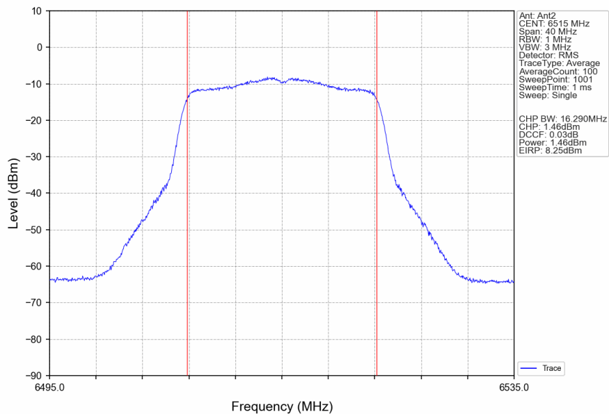
802.11a_HCH_6515MHz_Ant2_NTNV
