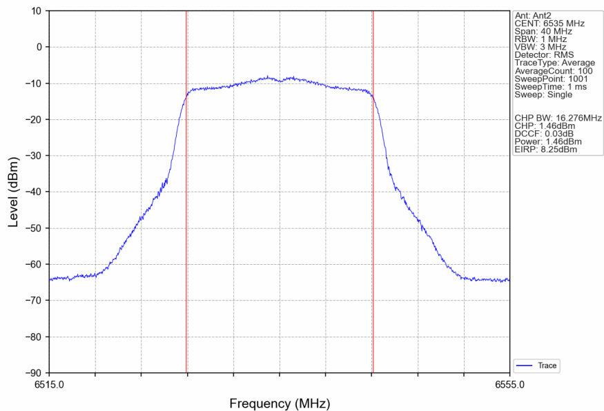
802.11a_LCH_6535MHz_Ant2_NTNV
