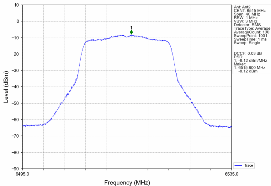
802.11a_HCH_6515MHz_Ant2_NTNV
