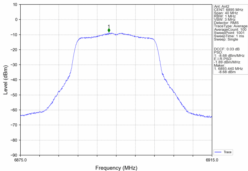
802.11a_LCH_6895MHz_Ant2_NTNV
