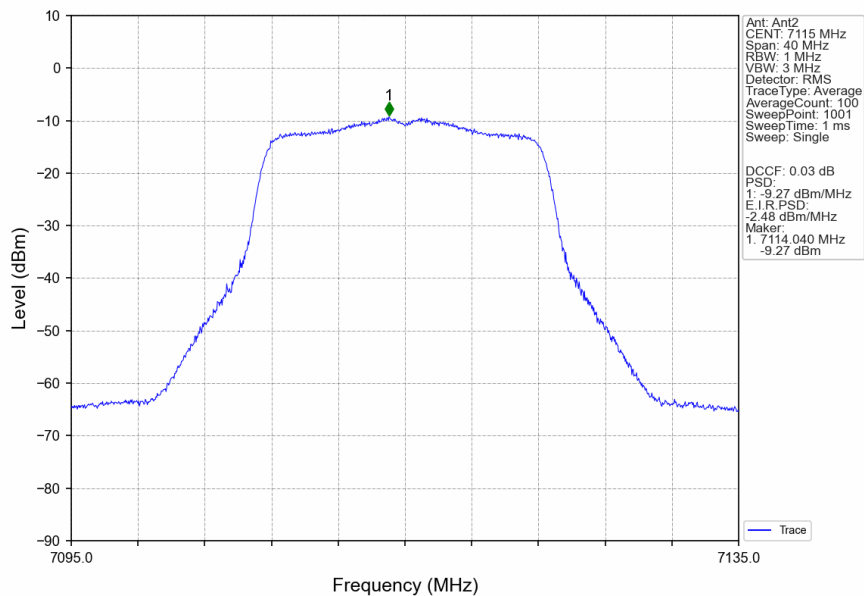
802.11a_HCH_7115MHz_Ant2_NTNV
