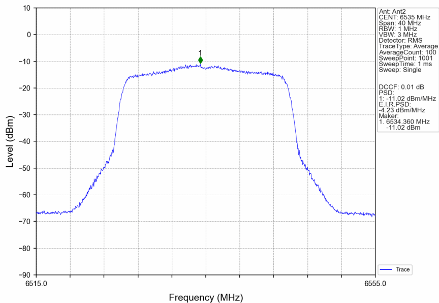
802.11ax(HEW20)_LCH_6535MHz_RU242_Left_Ant2_NTNV
