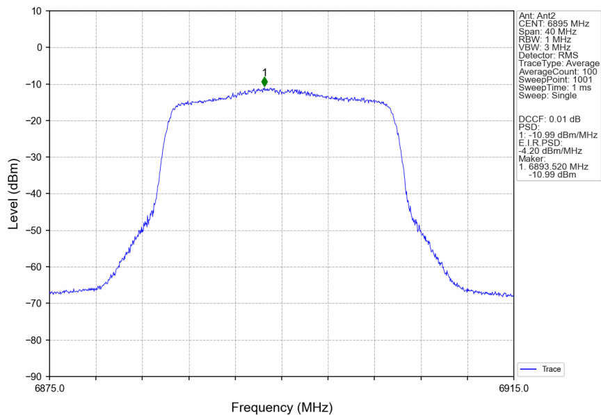
802.11ax(HEW20)_LCH_6895MHz_RU242_Left_Ant2_NTNV
