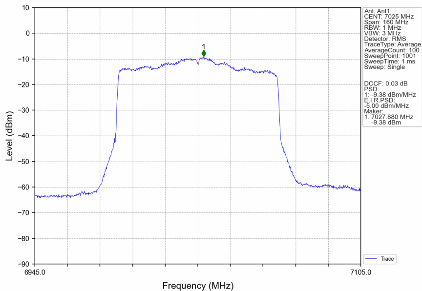
802.11ax(HEW80)_HCH_7025MHz_RU996_Left_Ant1_NTNV
