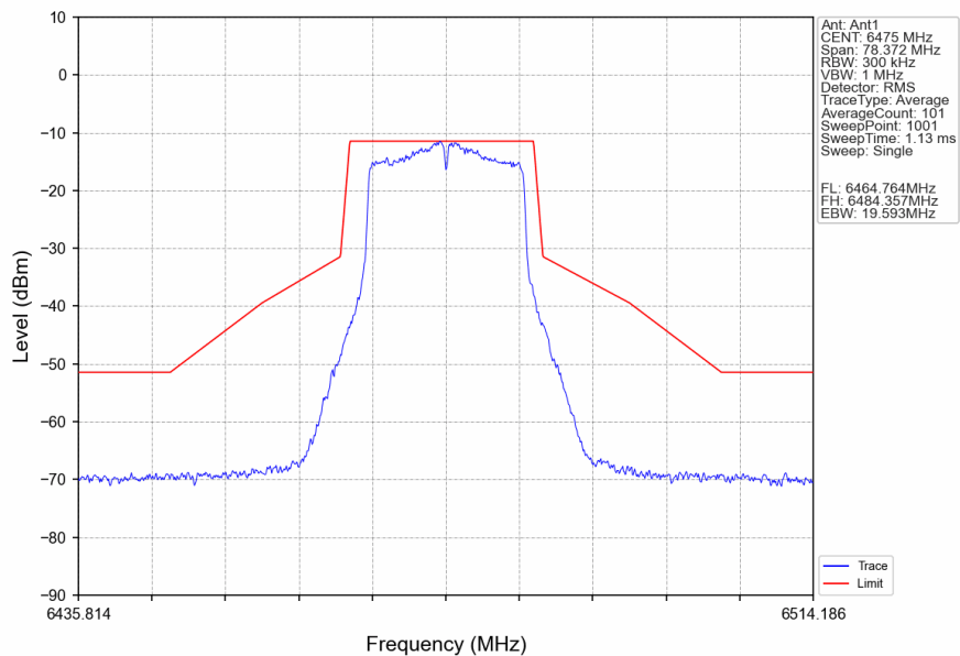
802.11a_MCH_6475MHz_Ant1_NTNV
