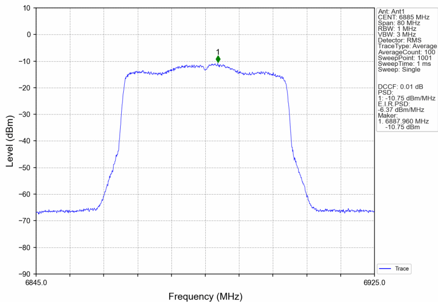
802.11ax(HEW40)_HCH_6885MHz_RU484_Left_Ant1_NTNV
