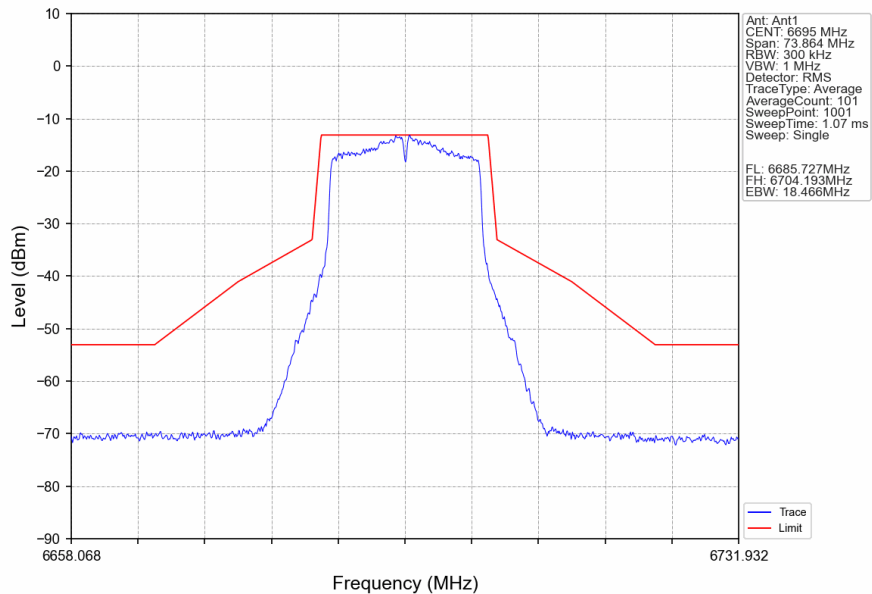
802.11a_MCH_6695MHz_Ant1_NTNV
