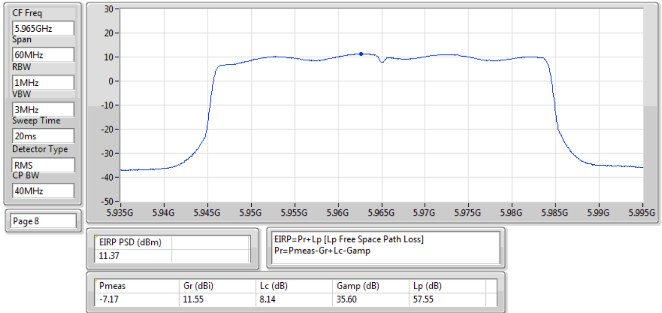
EIRP PSD;Band:6.2G;ax40;BWch:40MHz;Nss:1,(M0);Nant:2;Ch:5965MHz;TX
