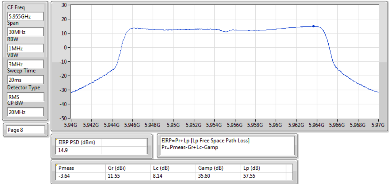
EIRP PSD;Band:6.2G;ax20;BWch:20MHz;Nss:1,(M0);Nant:2;Ch:5955MHz;TX
