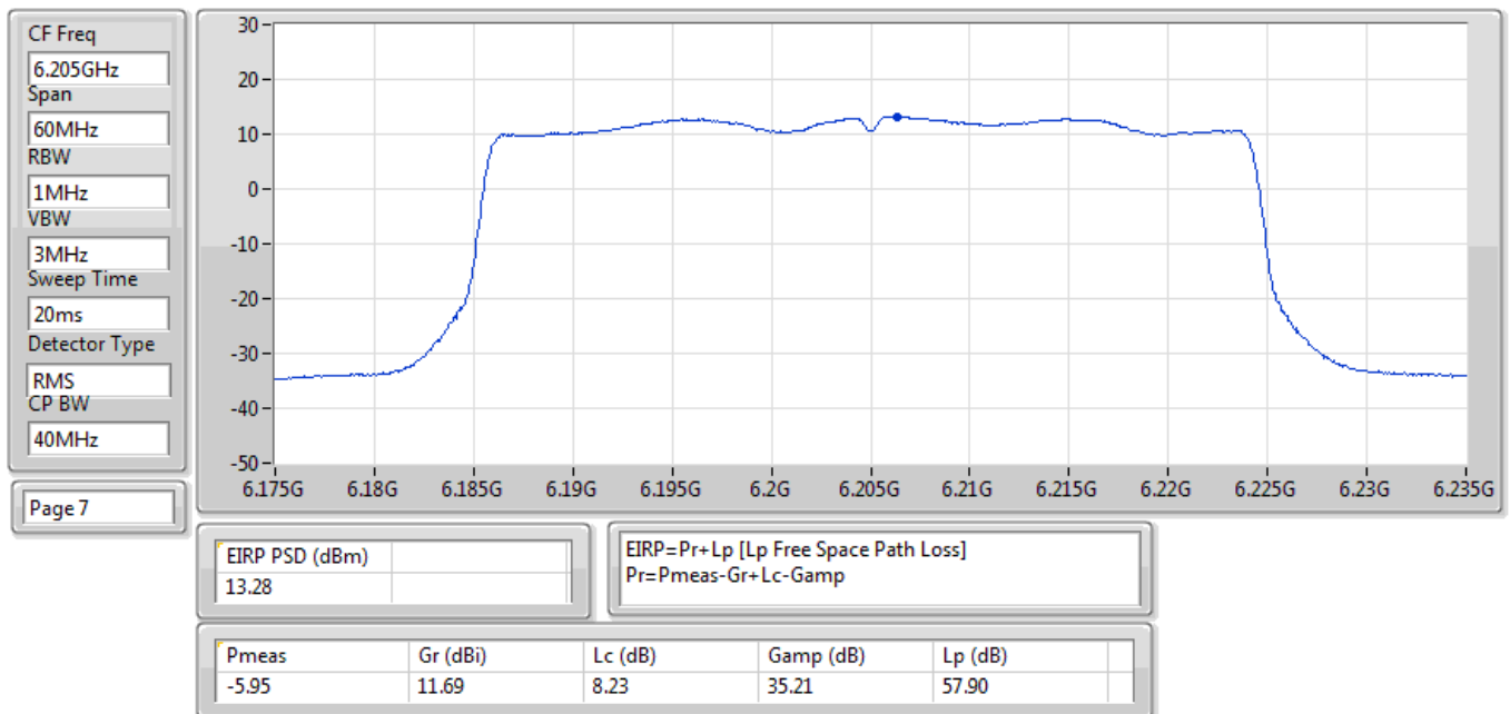
EIRP PSD;Band:6.2G;ax40;BWch:40MHz;Nss:1,(M0);Nant:2;Ch:6205MHz;TX
