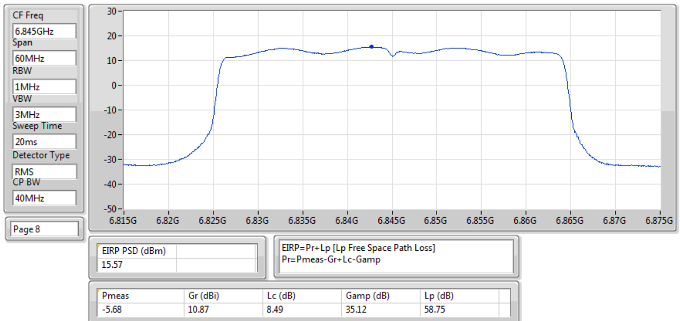
EIRP PSD;Band:6.7G;ax40;BWch:40MHz;Nss:1,(M0);Nant:2;Ch:6845MHz;TX
