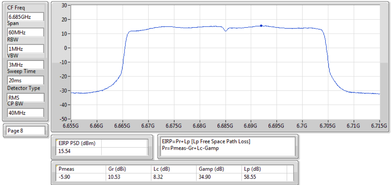
EIRP PSD;Band:6.7G;ax40;BWch:40MHz;Nss:1,(M0);Nant:2;Ch:6685MHz;TX
