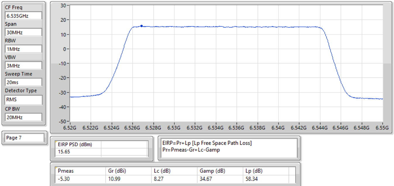
EIRP PSD; Band: 6.7G; QPSK; BWch: 20MHz; Nss: 1; Nant: 2; Ch: 6535MHz; TX
