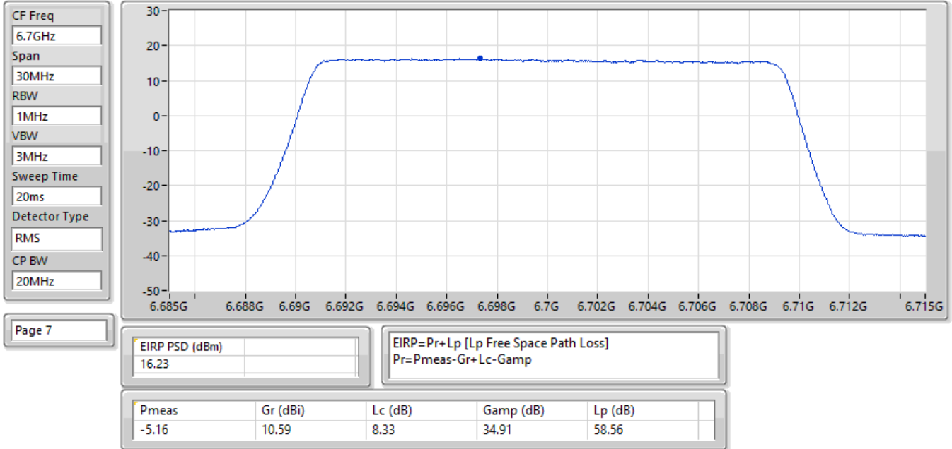
EIRP PSD; Band: 6.7G; QPSK; BWch: 20MHz; Nss: 1; Nant: 2; Ch: 6700MHz; TX
