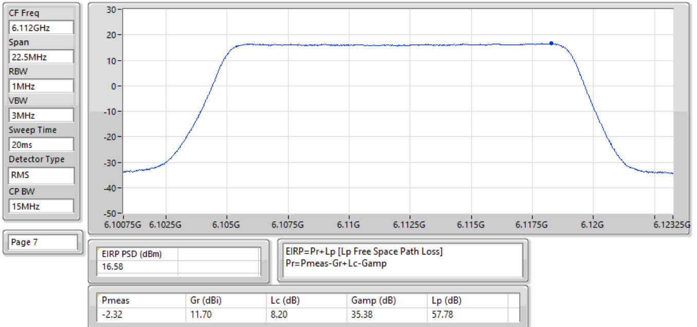
EIRP PSD;Band:6.2G;QPSK;BWch:15MHz;Nss:1;Nant:2;Ch:6112MHz;TX
