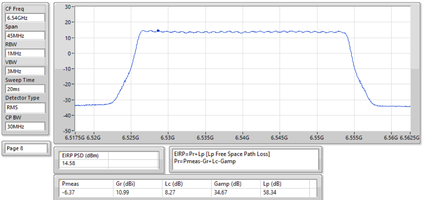
EIRP PSD; Band: 6.7G; QPSK; BWch: 30MHz; Nss: 1; Nant: 2; Ch: 6540MHz; TX
