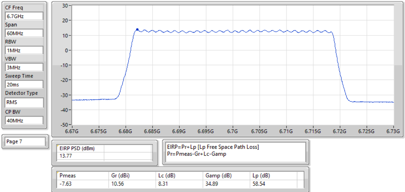
EIRP PSD; Band: 6.7G; QPSK; BWch: 40MHz; Nss: 1; Nant: 2; Ch: 6700MHz; TX
