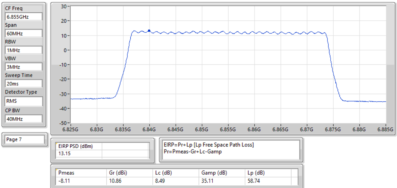
EIRP PSD; Band: 6.7G; QPSK; BWch: 40MHz; Nss: 1; Nant: 2; Ch: 6855MHz; TX
