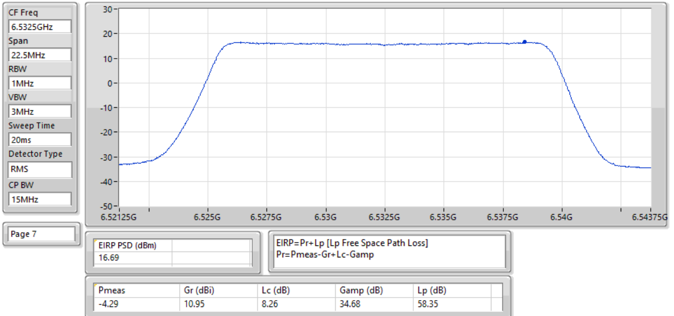
EIRP PSD;Band:6.7G;QPSK;BWch:15MHz;Nss:1;Nant:2;Ch:6532.5MHz;TX
