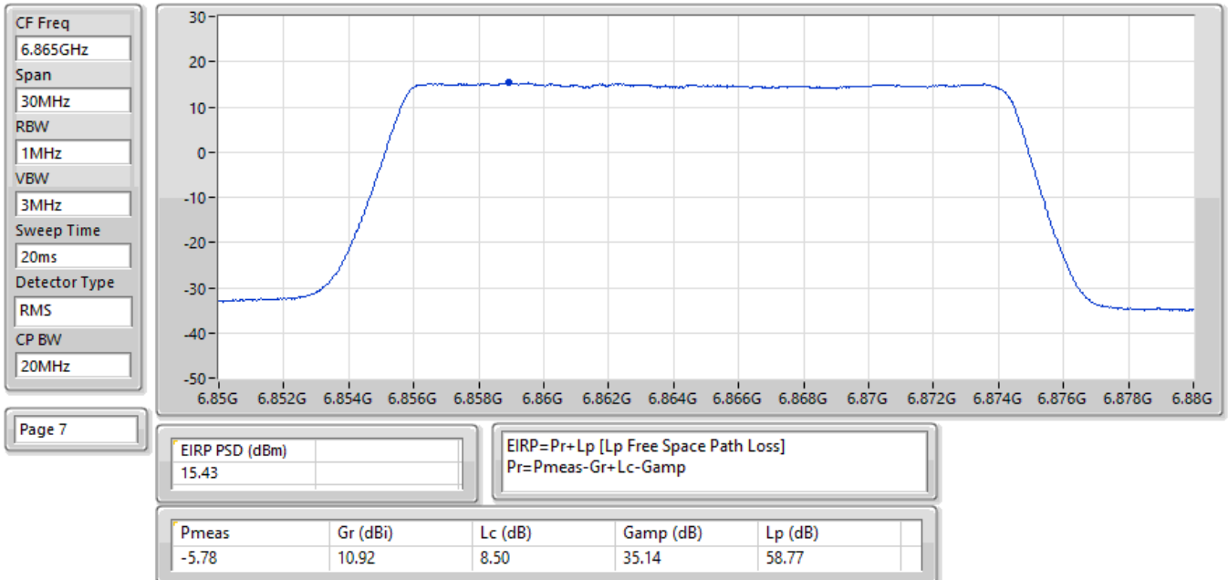
EIRP PSD; Band: 6.7G; QPSK; BWch: 20MHz; Nss: 1; Nant: 2; Ch: 6865MHz; TX
