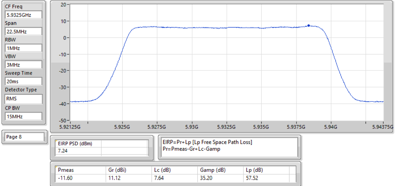
EIRP PSD;Band:6.2G;QPSK;BWch:15MHz;Nss:1;Nant:2;Ch:5932.5MHz;TX
