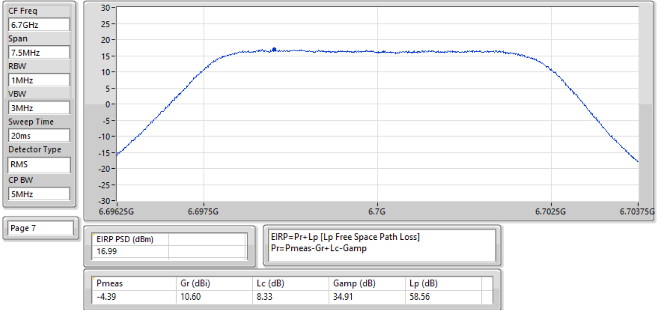
EIRP PSD;Band:6.7G;QPSK;BWch:5MHz;Nss:1;Nant:2;Ch:6700MHz;TX
