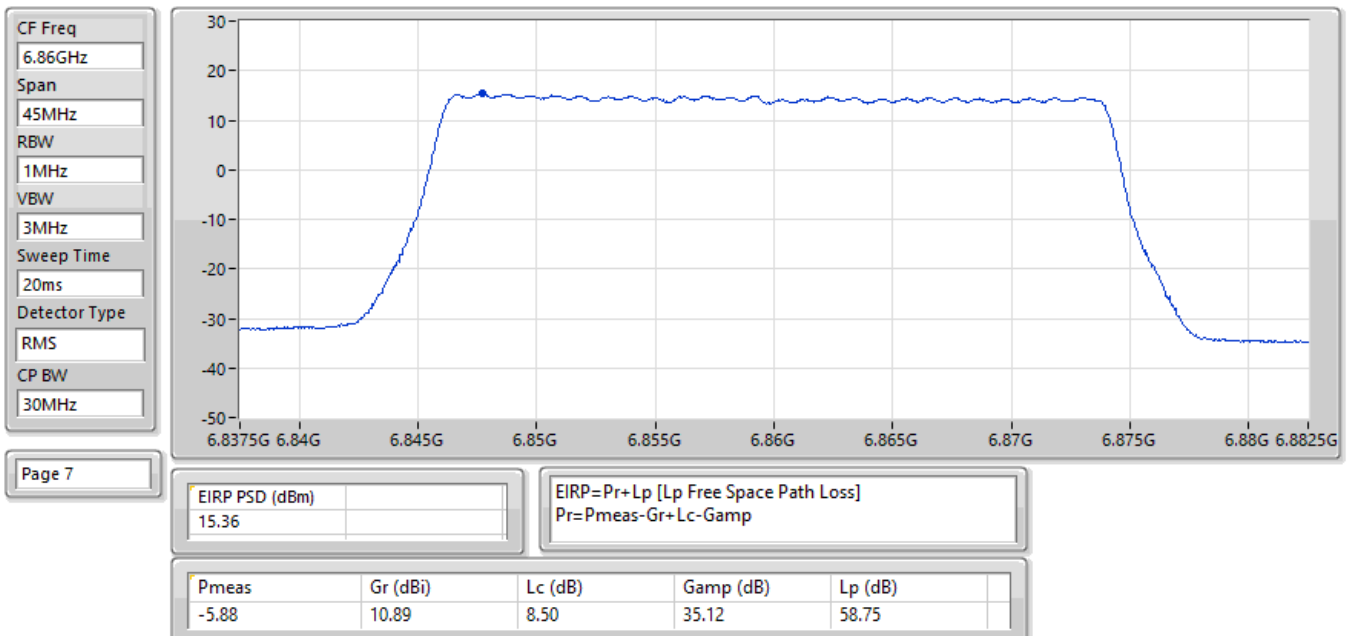
EIRP PSD; Band: 6.7G; QPSK; BWch: 30MHz; Nss: 1; Nant: 2; Ch: 6860MHz; TX
