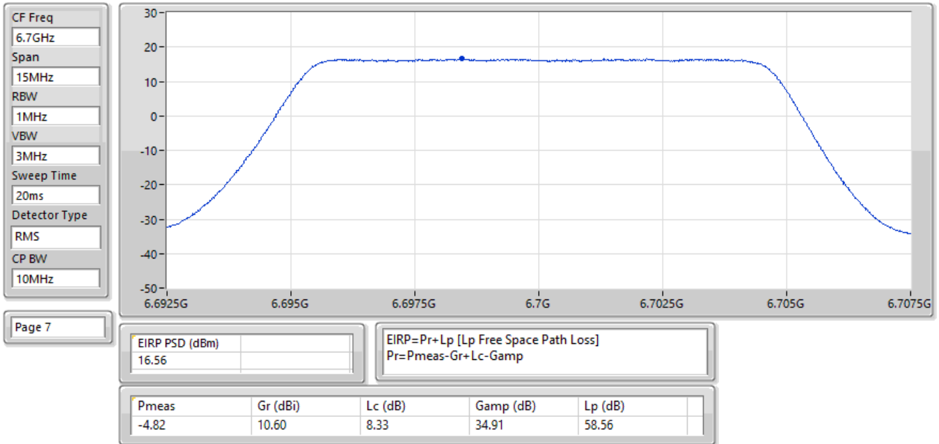
EIRP PSD; Band: 6.7G; QPSK; BWch: 10MHz; Nss: 1; Nant: 2; Ch: 6700MHz; TX
