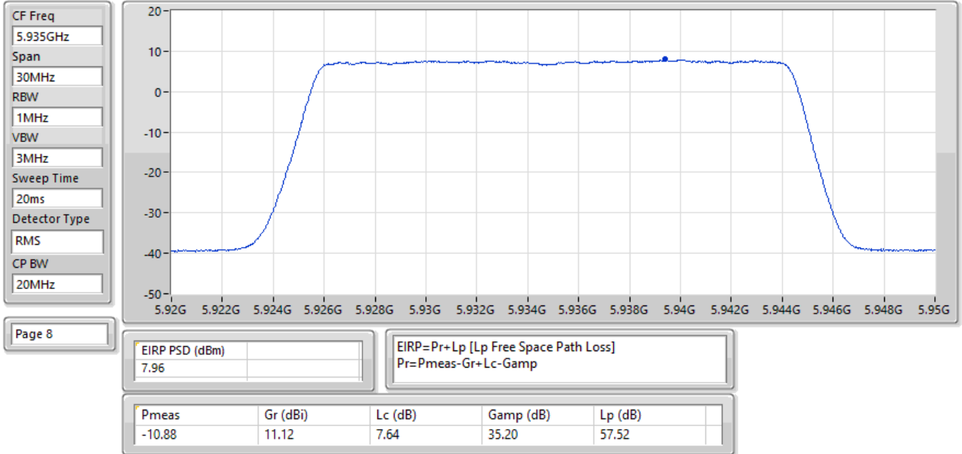
EIRP PSD; Band: 6.2G; QPSK; BWch: 20MHz; Nss: 1; Nant: 2; Ch: 5935MHz; TX
