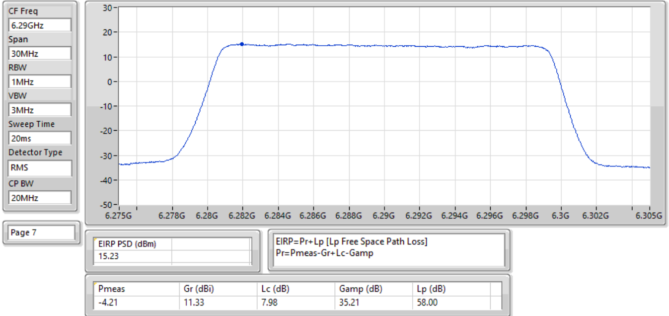
EIRP PSD; Band: 6.2G; QPSK; BWch: 20MHz; Nss: 1; Nant: 2; Ch: 6290MHz; TX
