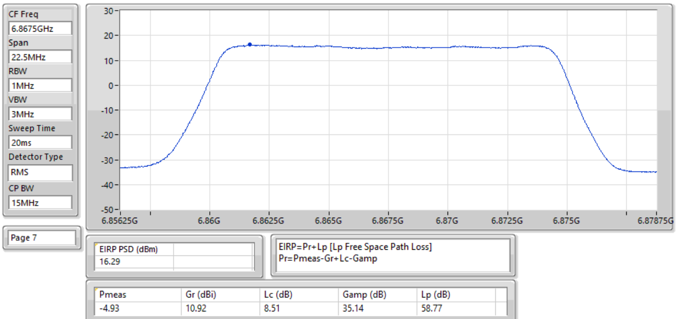
EIRP PSD;Band:6.7G;QPSK;BWch:15MHz;Nss:1;Nant:2;Ch:6867.5MHz;TX
