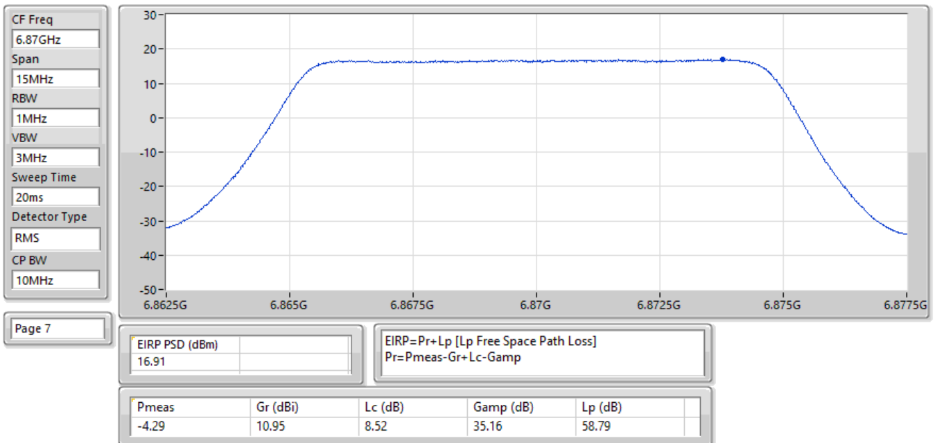
EIRP PSD; Band: 6.7G; QPSK; BWch: 10MHz; Nss: 1; Nant: 2; Ch: 6870MHz; TX
