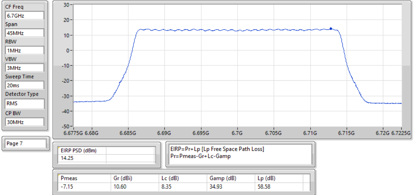
EIRP PSD; Band: 6.7G; QPSK; BWch: 30MHz; Nss: 1; Nant: 2; Ch: 6700MHz; TX
