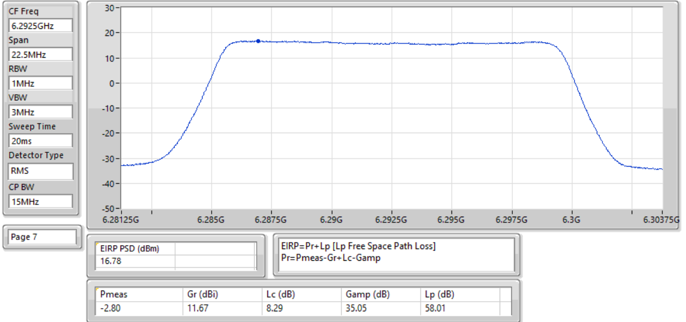
EIRP PSD;Band:6.2G;QPSK;BWch:15MHz;Nss:1;Nant:2;Ch:6292.5MHz;TX
