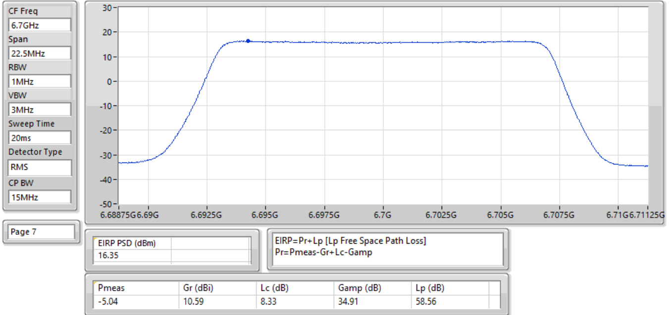
EIRP PSD;Band:6.7G;QPSK;BWch:15MHz;Nss:1;Nant:2;Ch:6700MHz;TX
