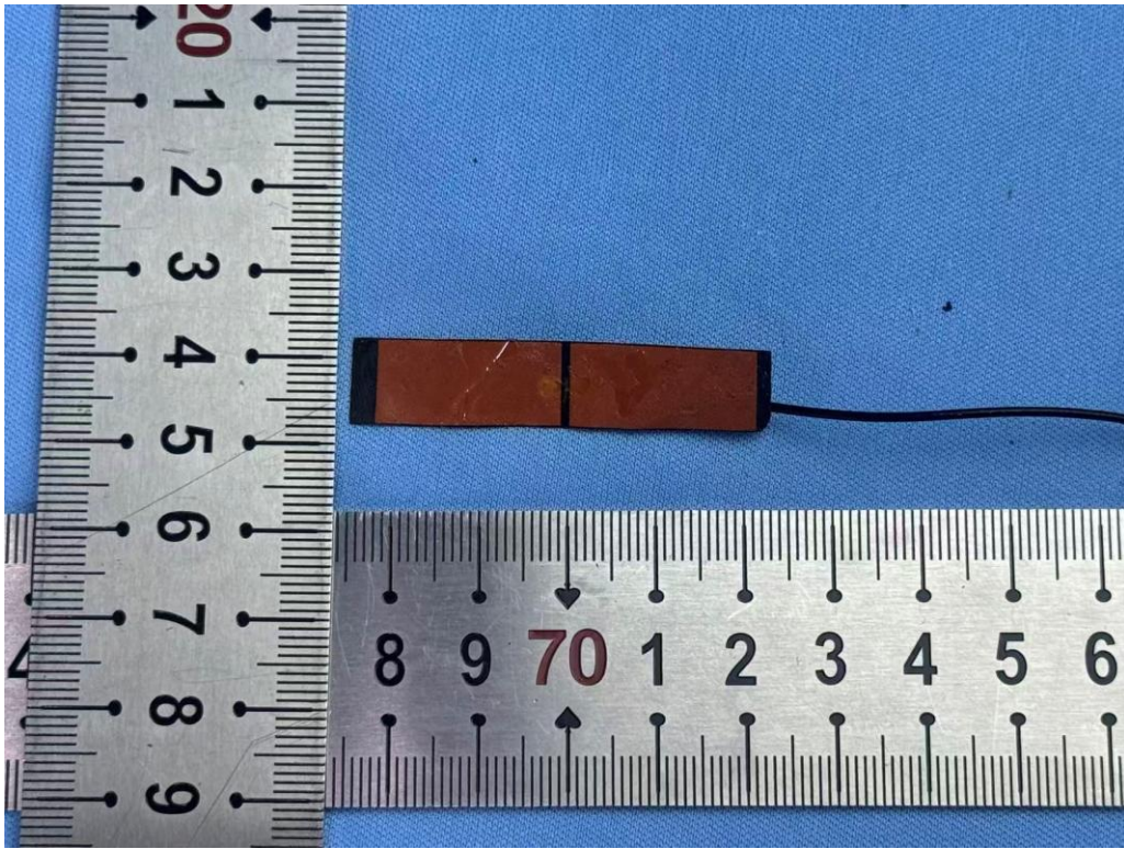
2.4GHz ANT
