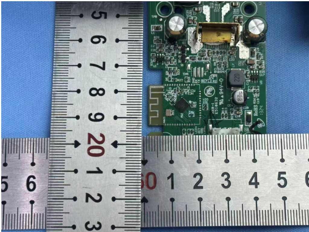
2.4GHz ANT
