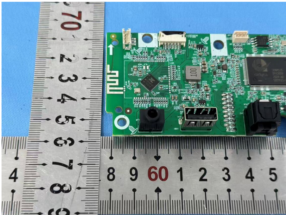
BT ANT
