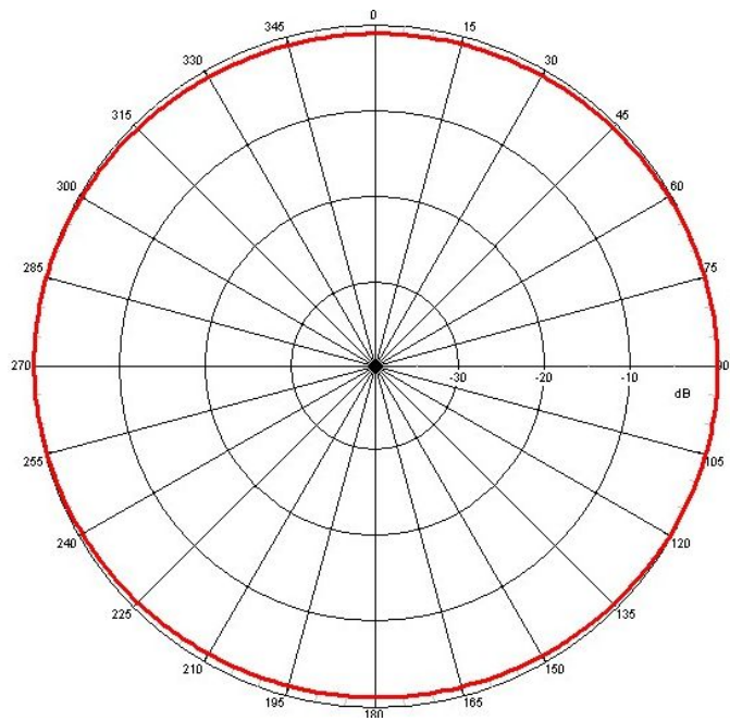
H-PLANE
