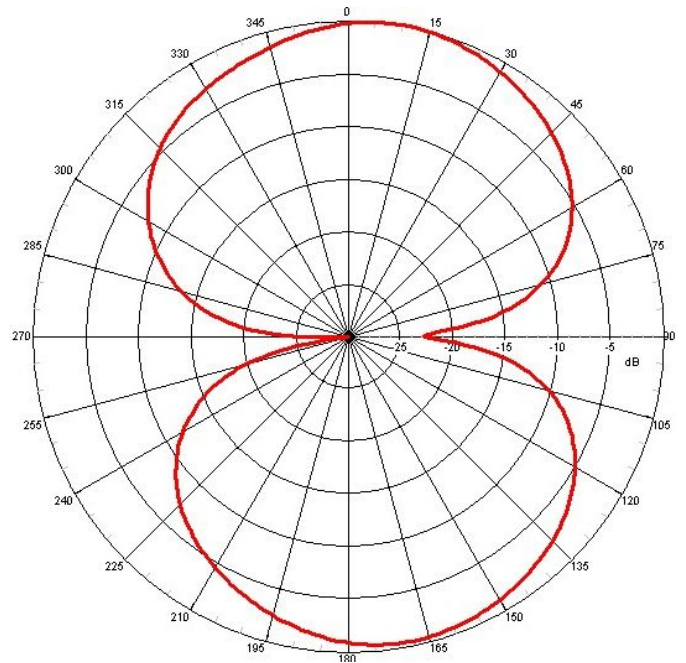
E-PLANE
