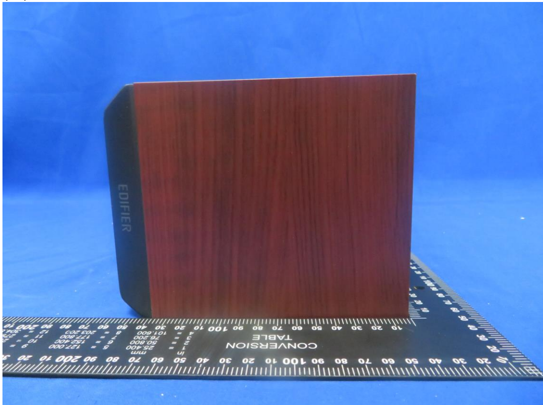
(12) EUT Photo
