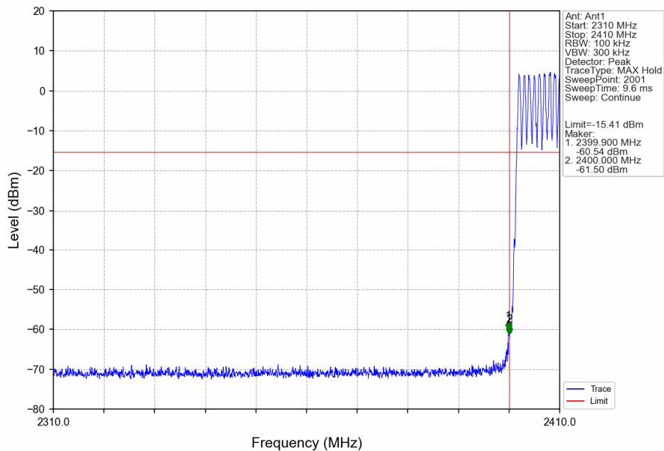
GFSK_DH5_HOPP_2400MHz_Ant1_NTNV
