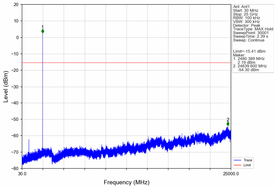
GFSK_DH5_HOPP_2400MHz_Ant1_NTNV
