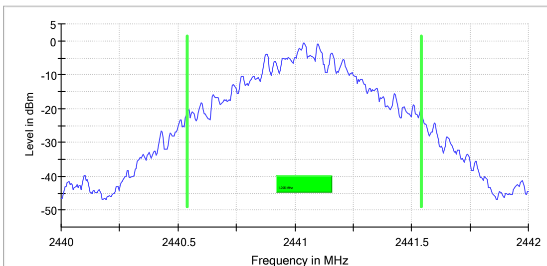
DH5_Ant1_2441
