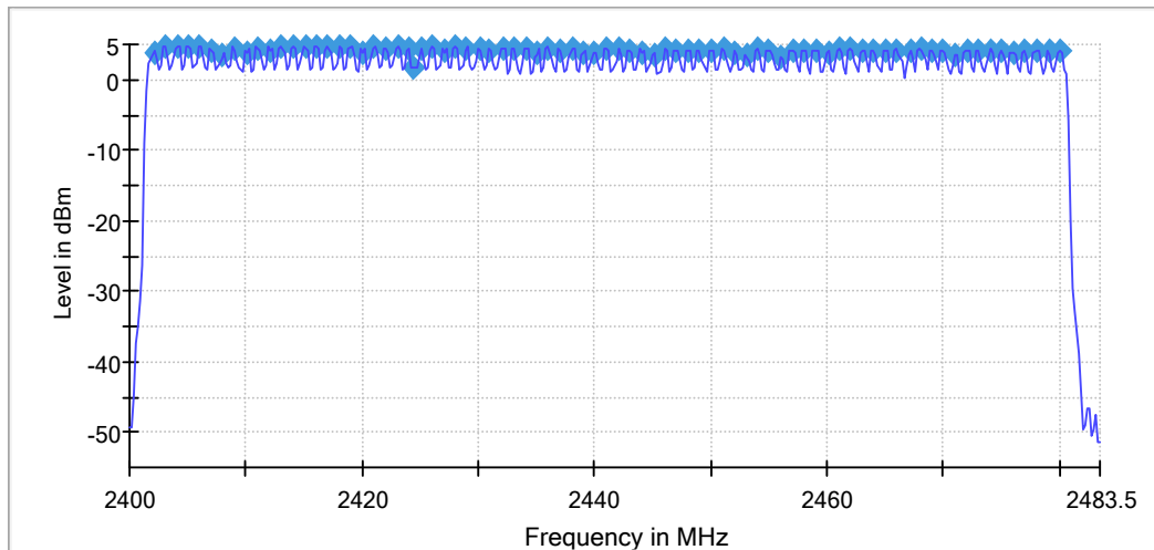
2DH5_Ant1_Hop
