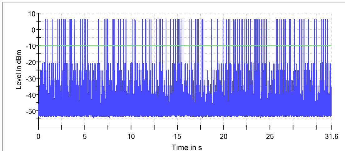
2DH5_Ant1_Hop
