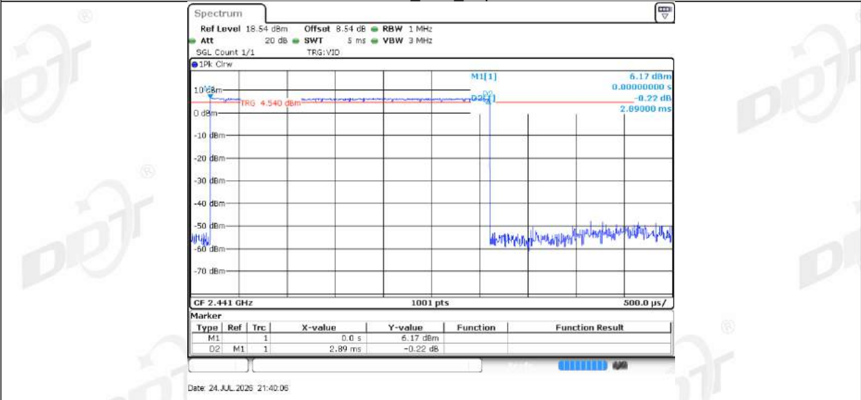
2DH5_Ant1_Hop
