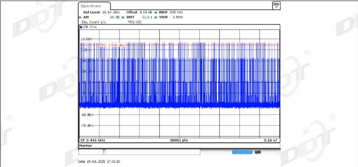
2DH5_Ant1_Hop
