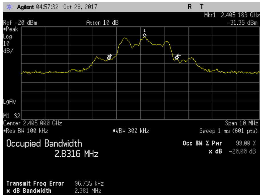
Figure 7.2.2-1: 20dB / 99% BW
