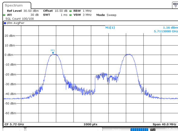
ax20_5720MHz_RU_26/8_Chain 1
