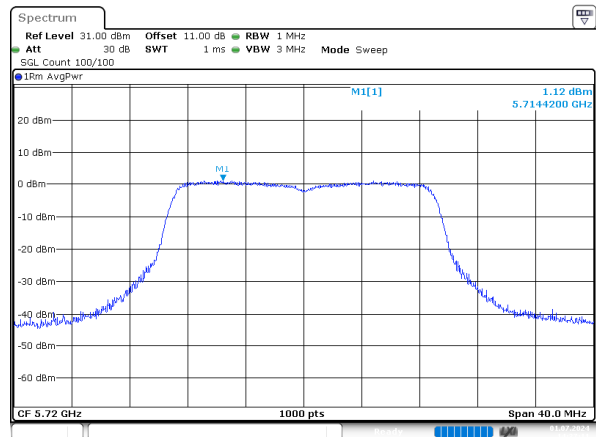
ac20_5720MHz_Chain 1
