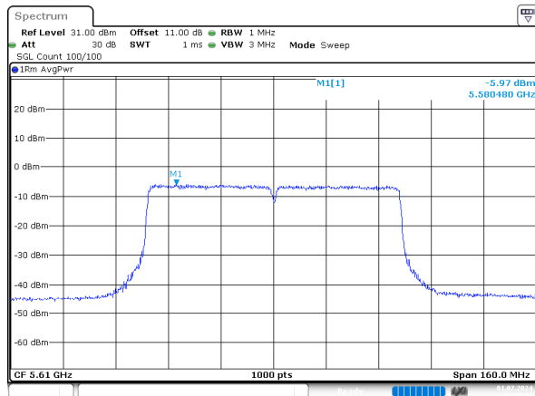
ac80_5610MHz_Chain 0
