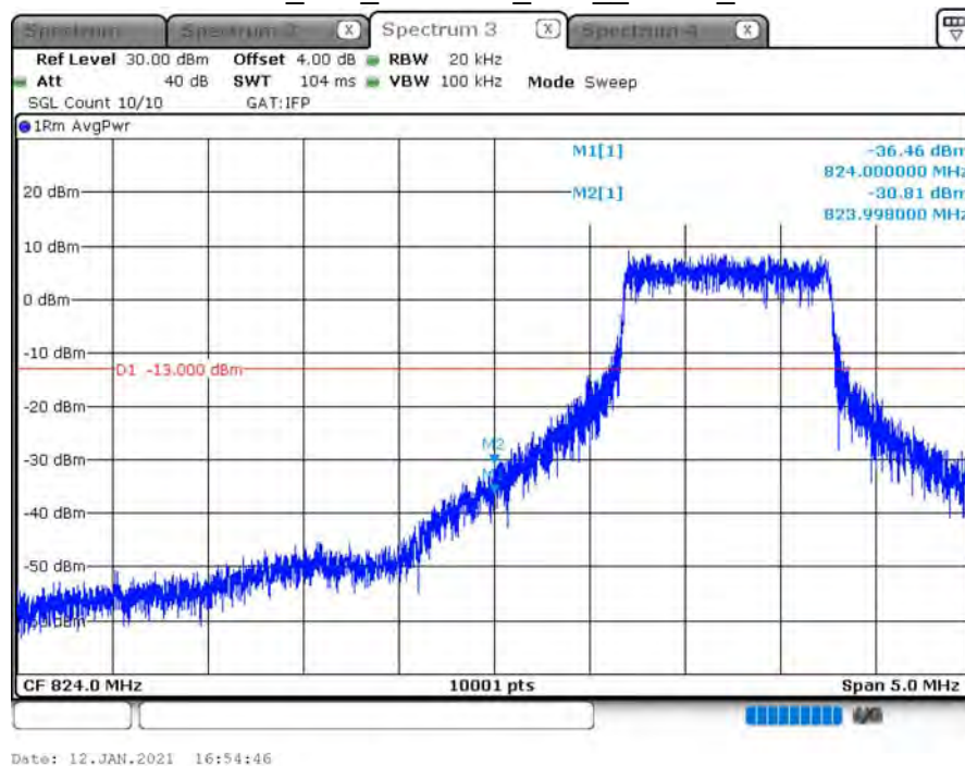
CAT-M1_B26_CH26840_10M_QPSK_6RB0
