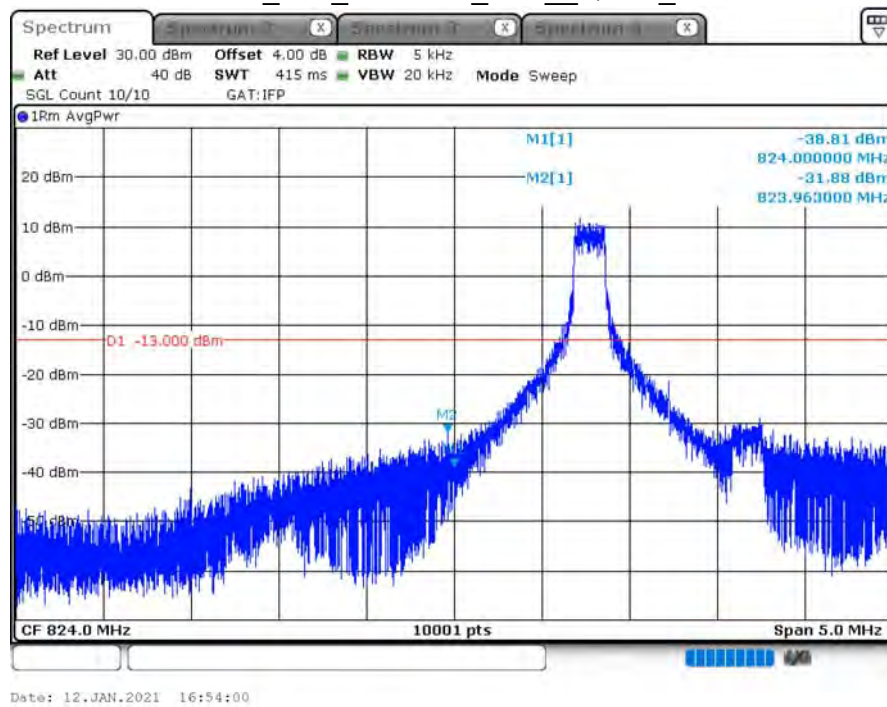
CAT-M1_B26_CH26840_10M_QPSK_1RB0
