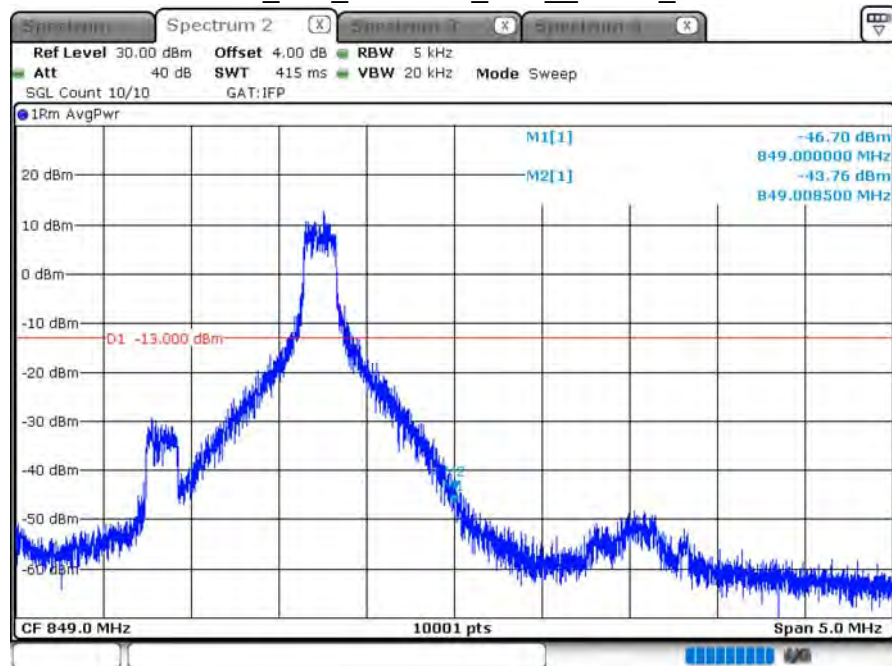
CAT-M1_B26_CH26990_10M_QPSK_1RB5
