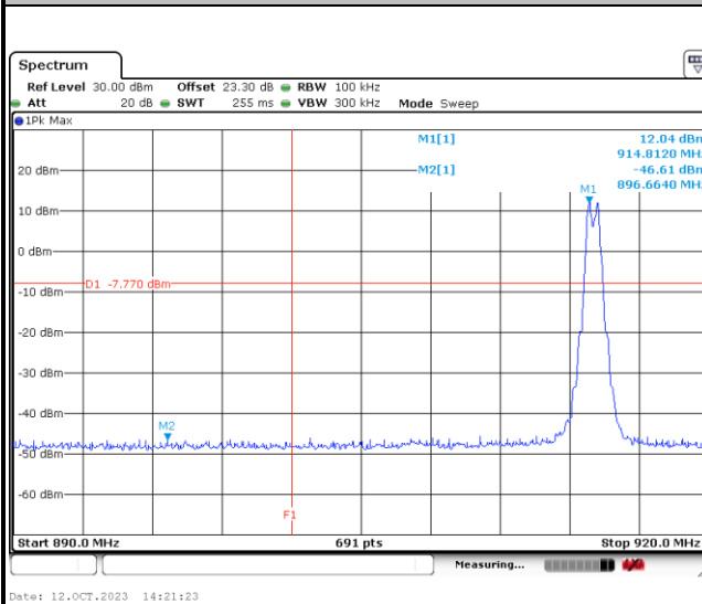
Band Edge Plot
