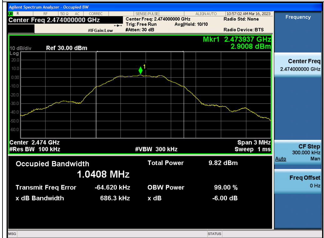
Test_Graph_GFSK_ANT1_2474_DTSBW
