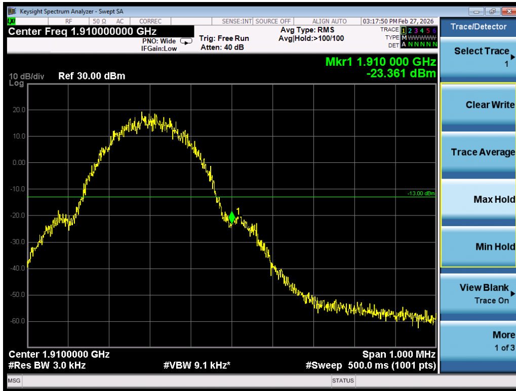
Band edge\GSM1900\GPRS\H
