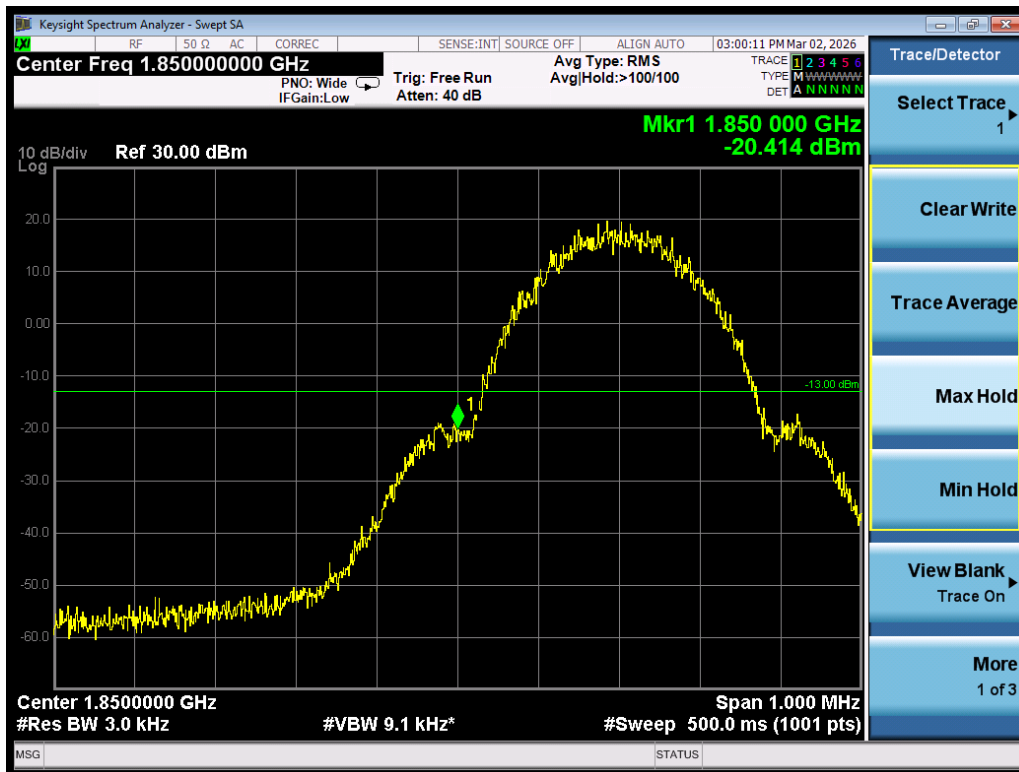
Band edge\GSM1900\GSM\L
