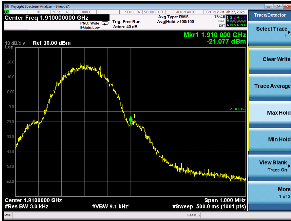
Band edge\GSM1900\GSM\H
