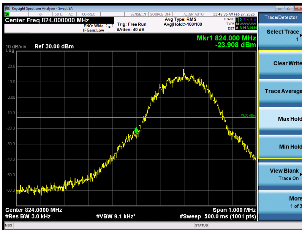
Band edge\GSM850\EGPRS\L
