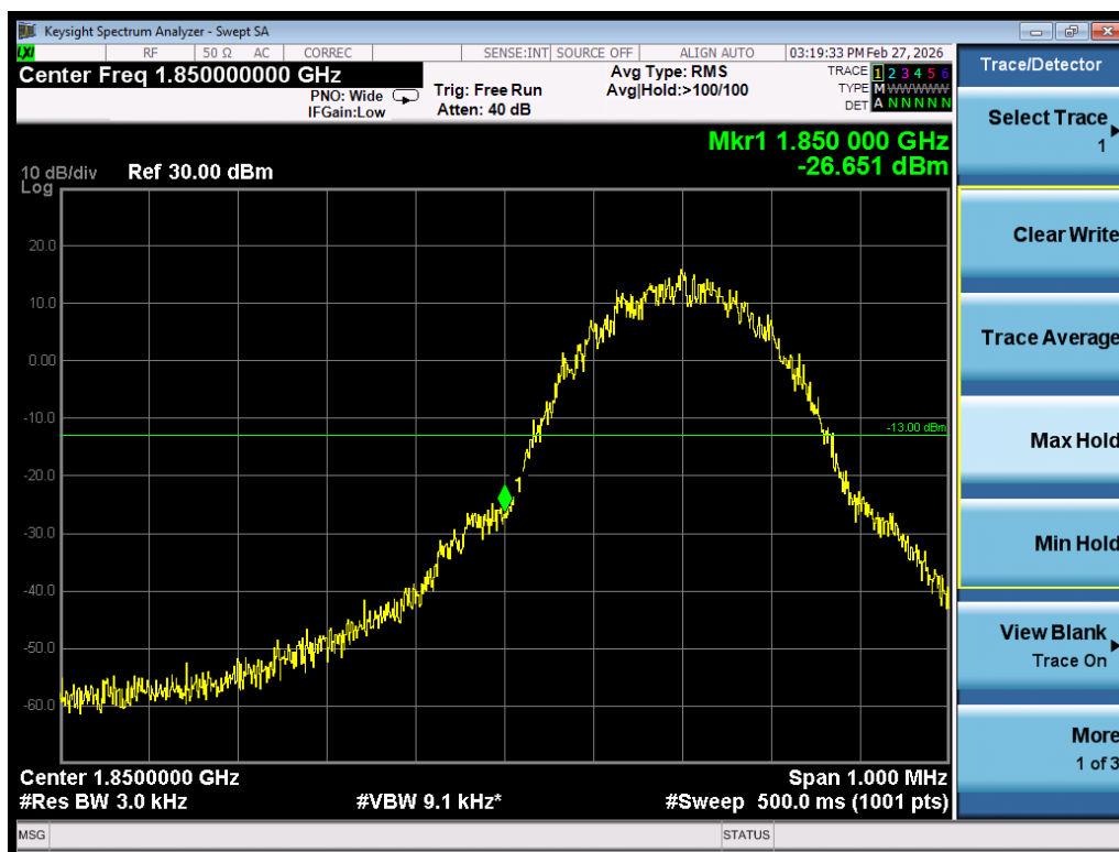
Band edge\GSM1900\EGPRS\L
