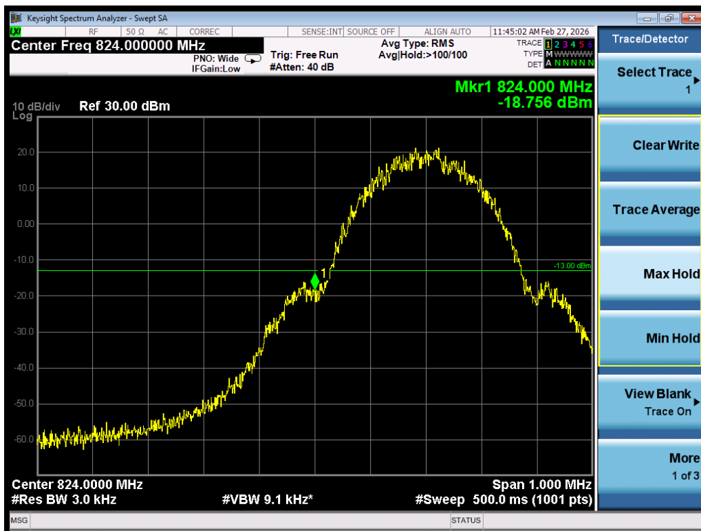
Band edge\GSM850\GPRS\L
