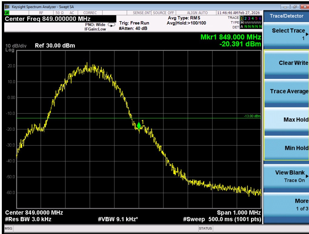
Band edge\GSM850\GPRS\H
