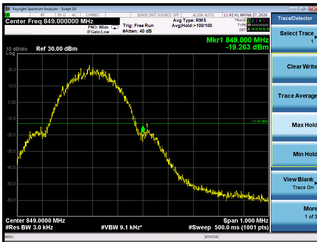
Band edge\GSM850\GSM\H
