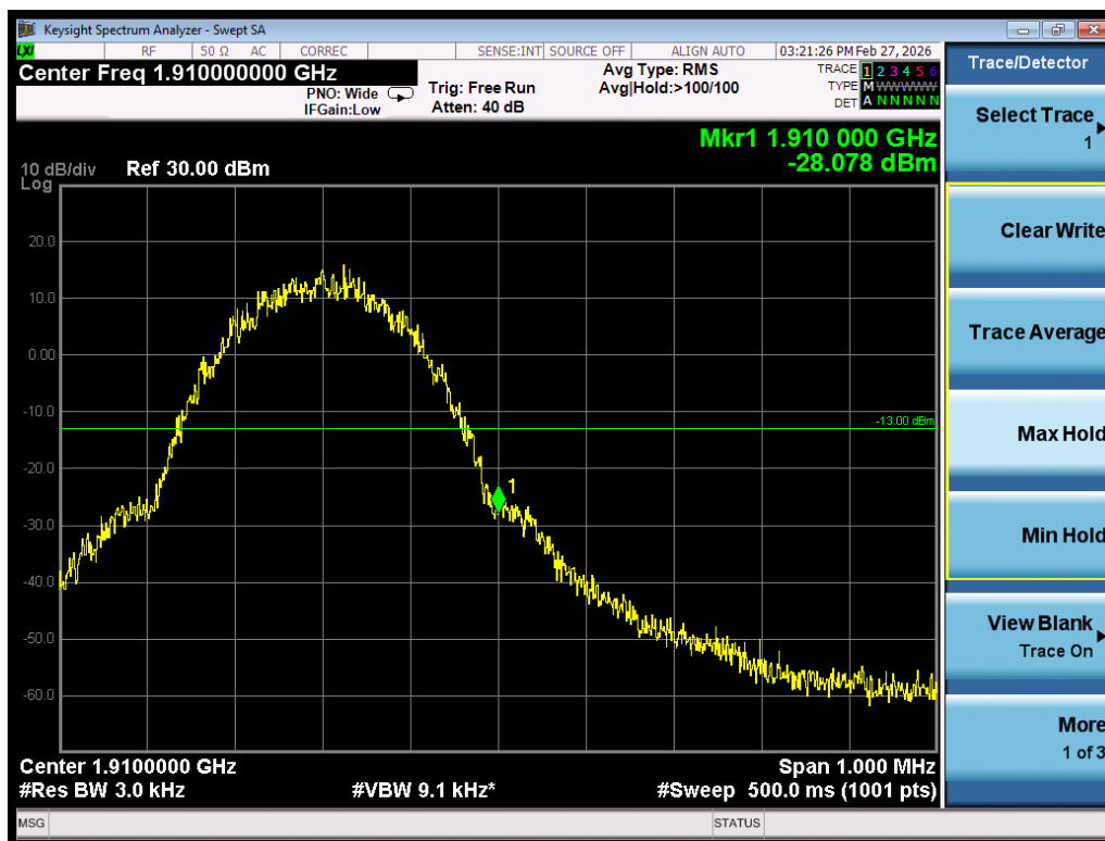
Band edge\GSM1900\EGPRS\H
