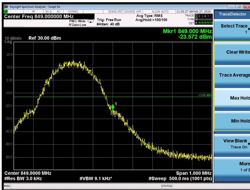
Band edge\GSM850\EGPRS\H
