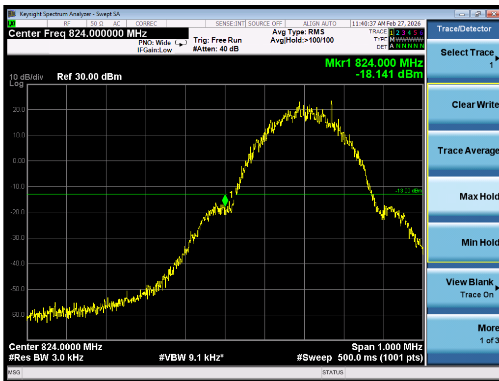
Band edge\GSM850\GSM\L
